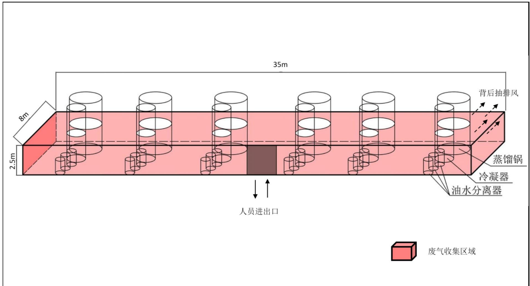
图 8.2-1 (b) 本项目废气收集区域示意图
