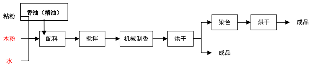
图 6.1-1 不同香型卫生香生产工艺流程图
