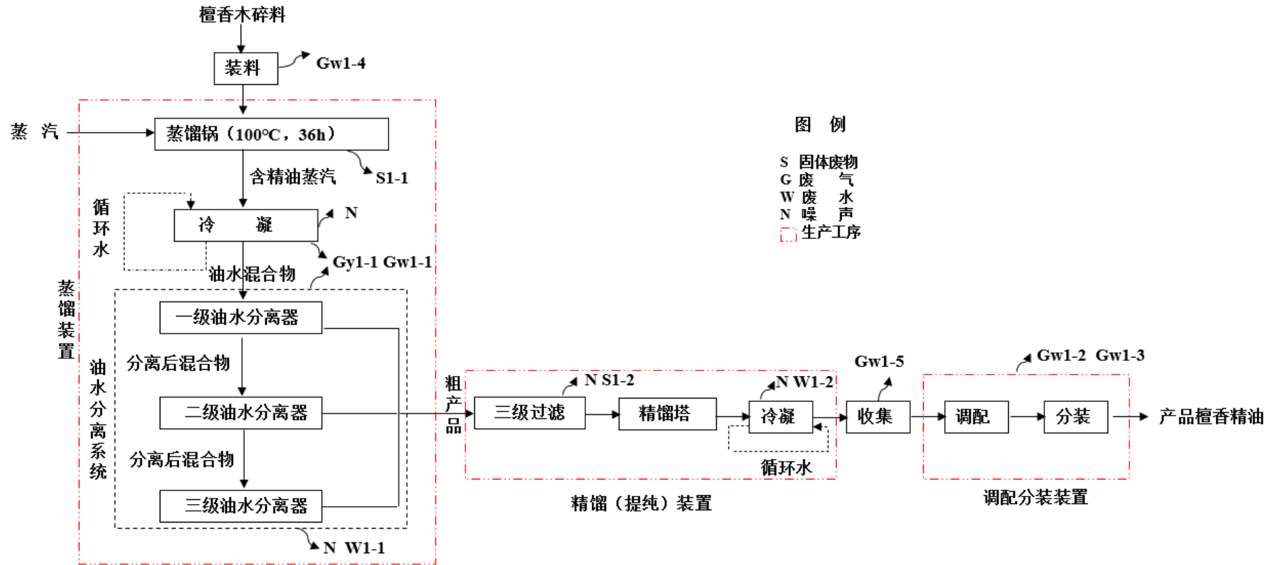
图 3.4-2 檀香精油生产工艺流程及产污环节示意图
