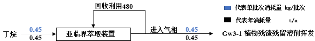
图 3.5-8 丁烷物料平衡分析图 单位 kg/批次 (t/a)
