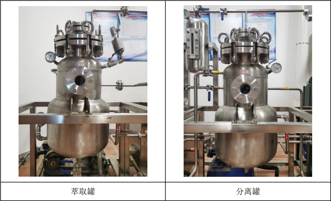
亚临界萃取实验室成套设备
