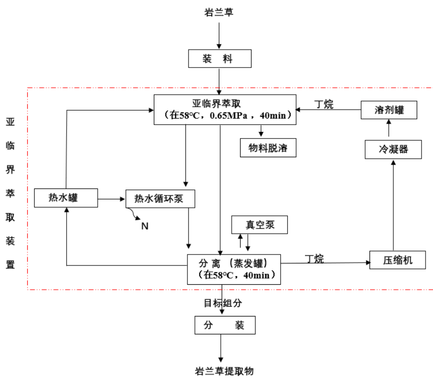
图 3.1-13 亚临界萃取装置工艺流程图
