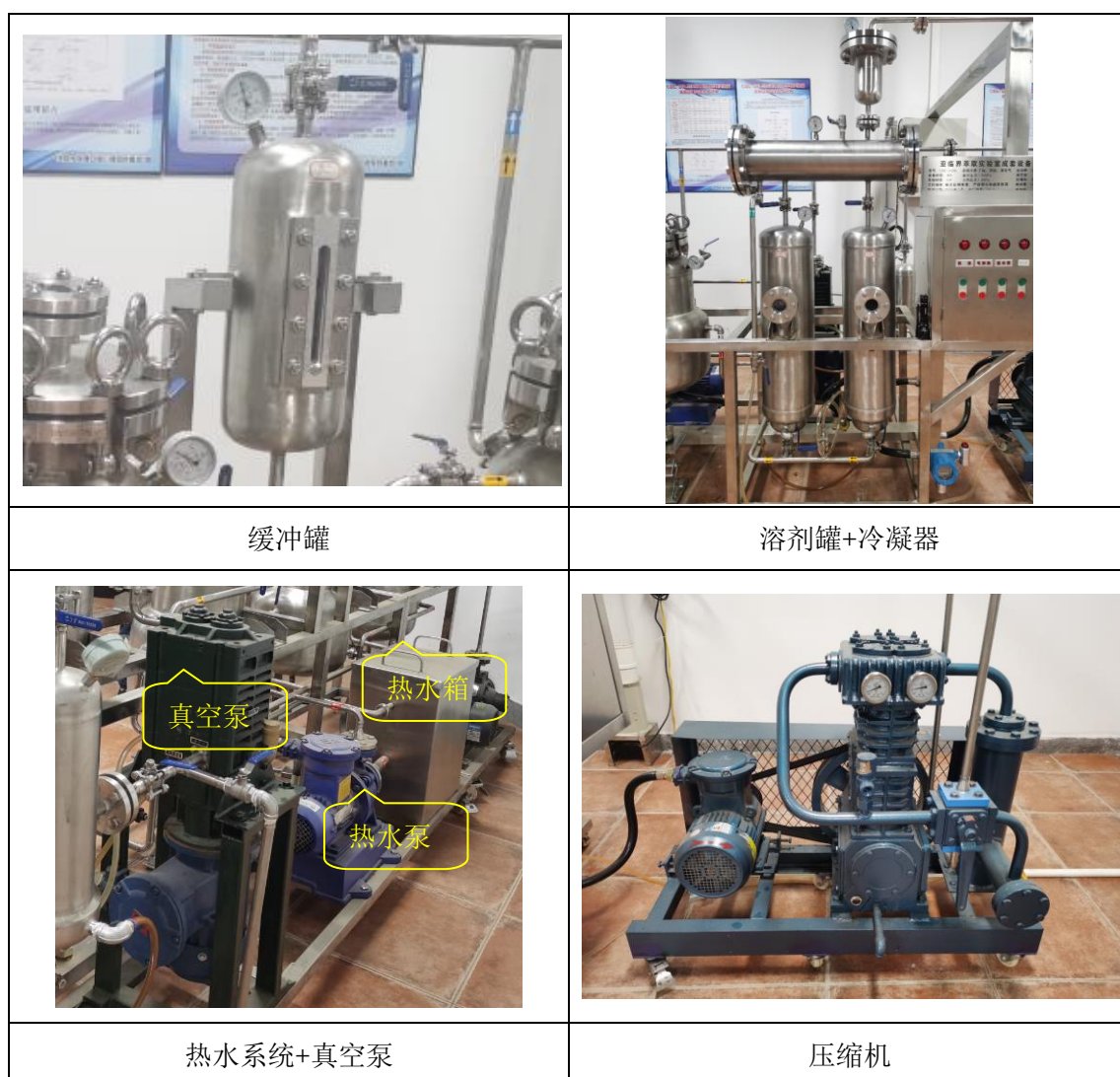
图 3.1-12 亚临界萃取实验室成套设备照片
