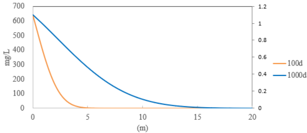
图 6.5-1 污染物 COD Cr 连续渗漏情况预测统计图
