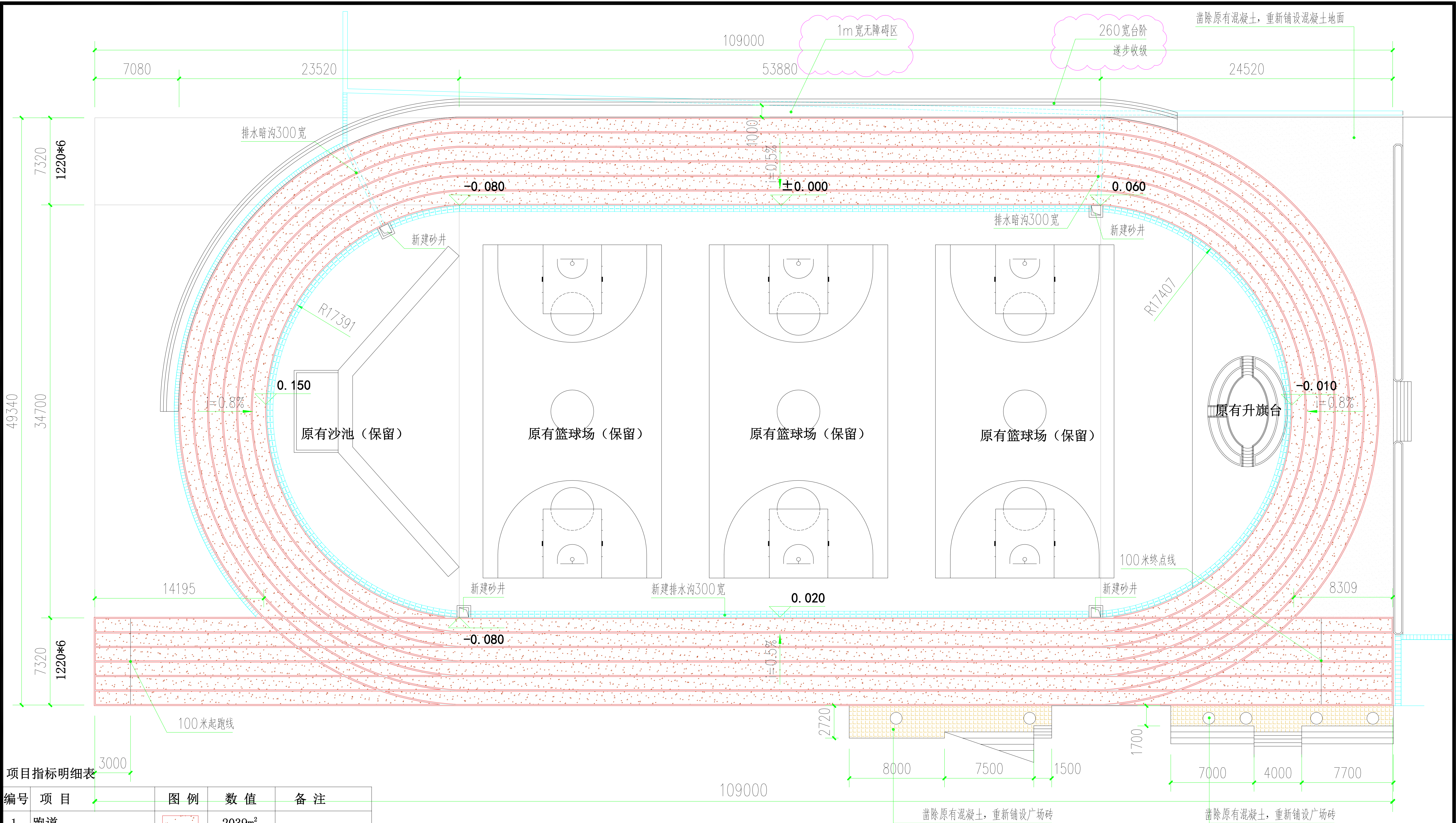
塑胶运动场平面图 1:300
