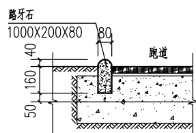
路牙石做法大样
