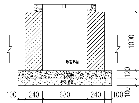
2-2剖面图
