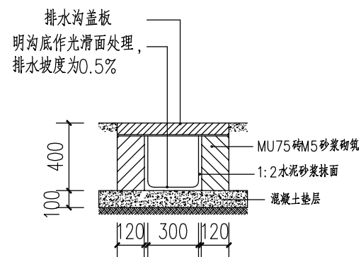
排水沟做法大样
