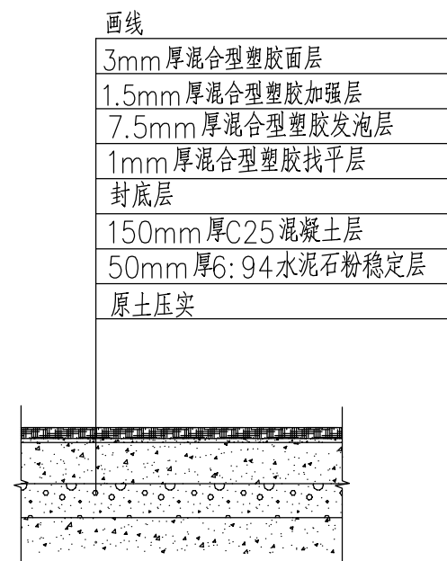
跑道做法大样
