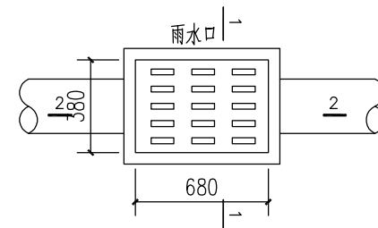
砂井（雨水进水井）平面图
