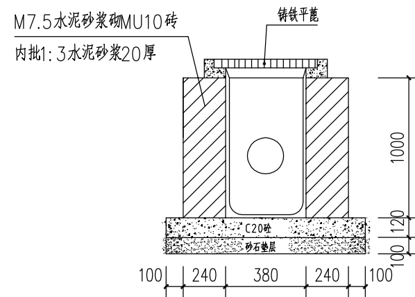
1-1剖面图
