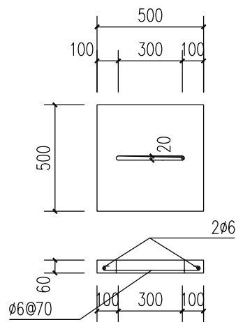
排水沟盖板大样 1:100
