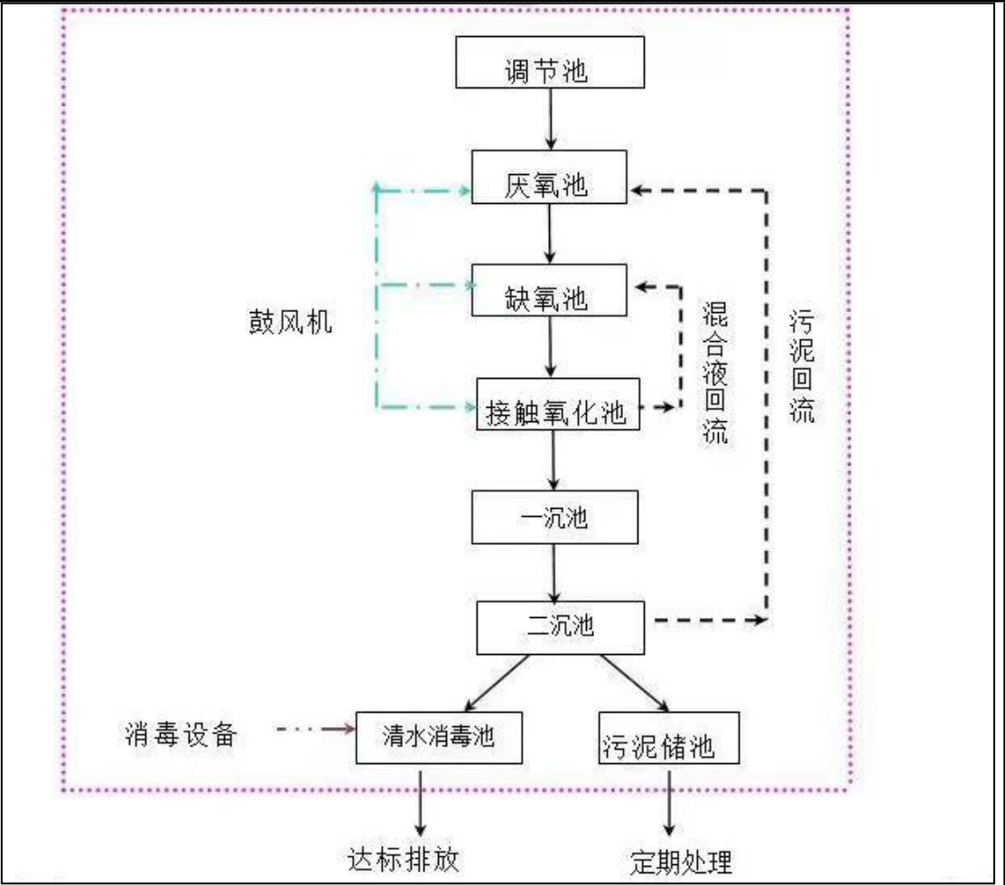
图 4-1 银洲湾科创产业园配套污水处理厂污水处理流程图
