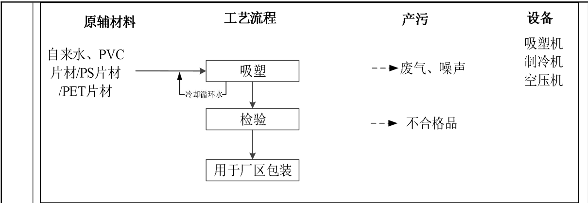
图 2-3 塑料包装材料吸塑加工工艺流程图（厂内使用）
