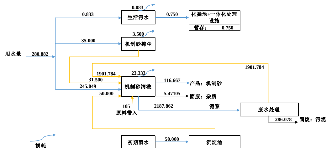
图2. 项目雨季水平衡图 (m³/d)
