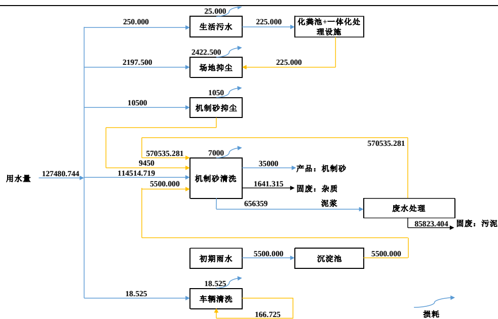
图3. 项目总水平衡图 (m³/a)
