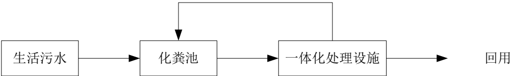
图6. 生活污水处理工艺
