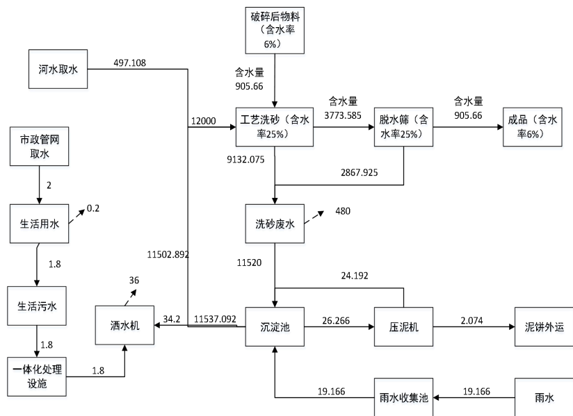
图 2-2 改扩建后汛期（丰水期）时水平衡图 单位：m³/d
