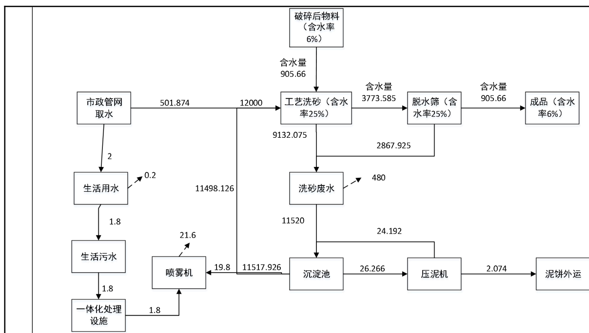
图 2-9 现有项目非汛期（枯水期）水平衡图 单位：m³/d
