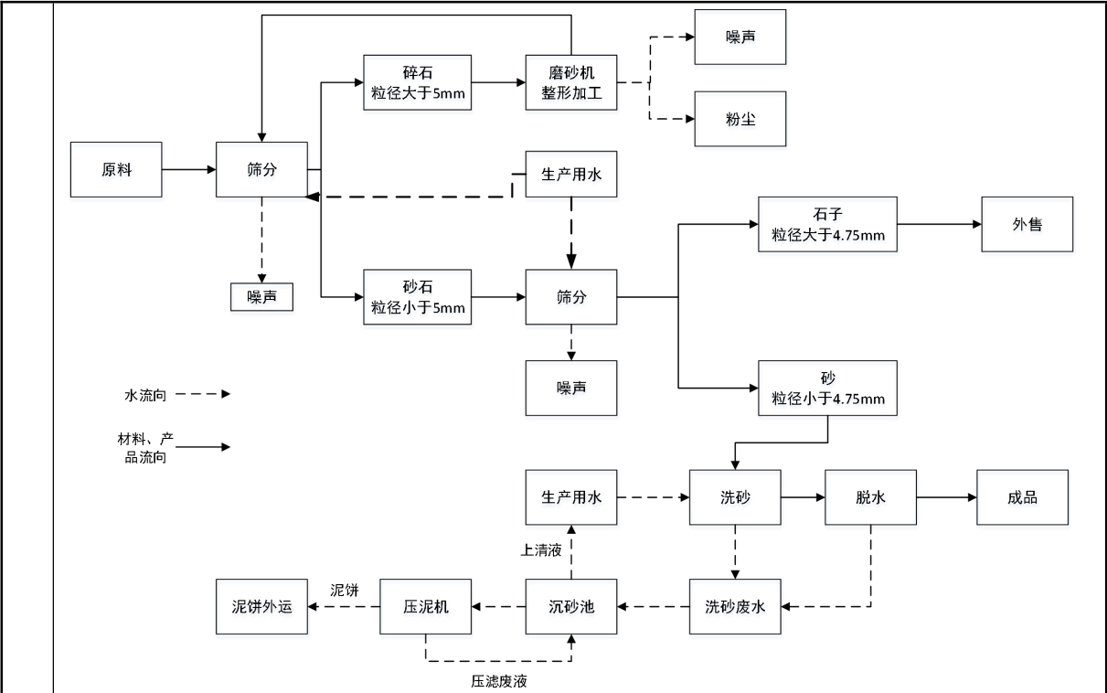
图 2-5 营运期机制砂生产线工艺流程图
