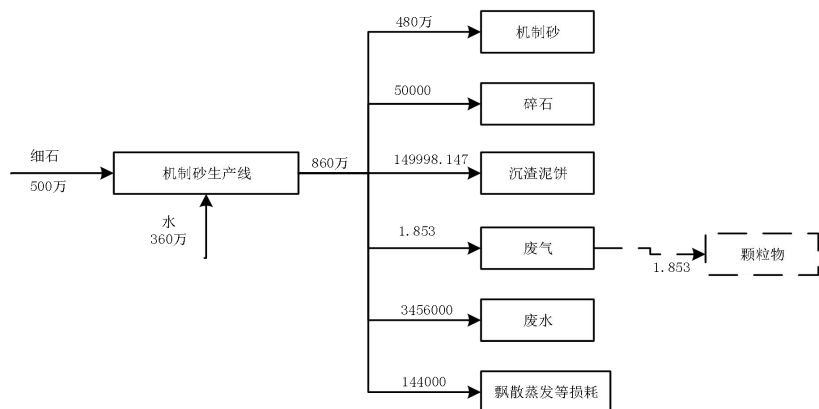
图 2-1 生产项目物料平衡图 单位：t/a
