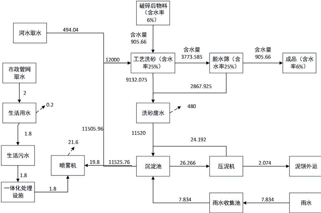
图 2-8 现有项目汛期（丰水期）水平衡图 单位：m³/d
