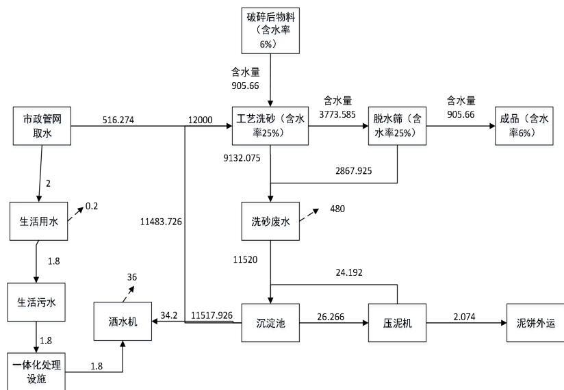
图 2-3 改扩建后非汛期（枯水期）时水平衡图 单位：m³/d
