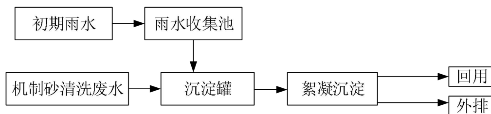
图 6.2-2 生产废水处理工艺流程图
