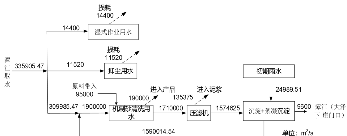
图 2.2-1 项目生产过程水平衡图
