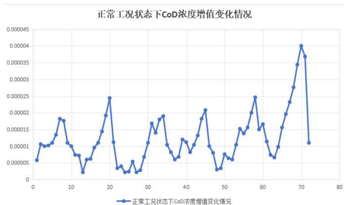
图 5.2-6 正常排放情况排污口区域 COD 浓度增值变化情况
