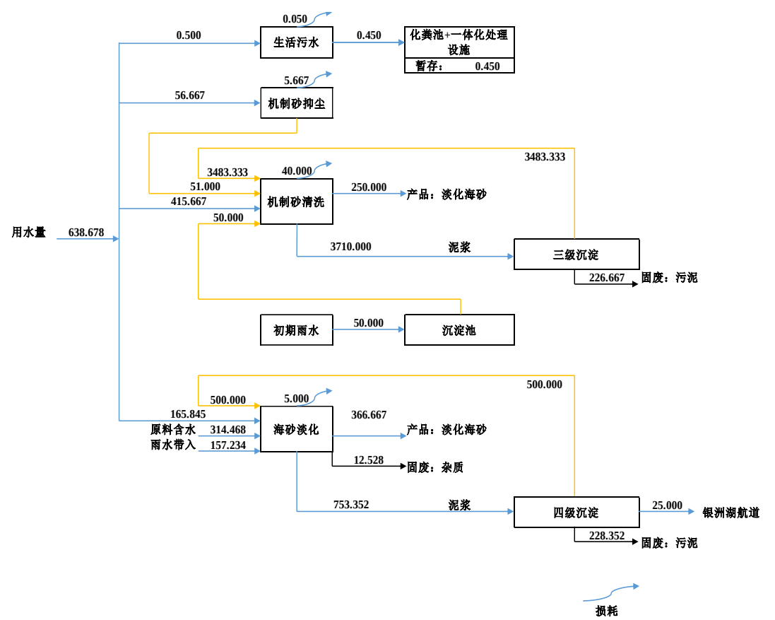
图2. 项目雨季水平衡图 (m³/d)
