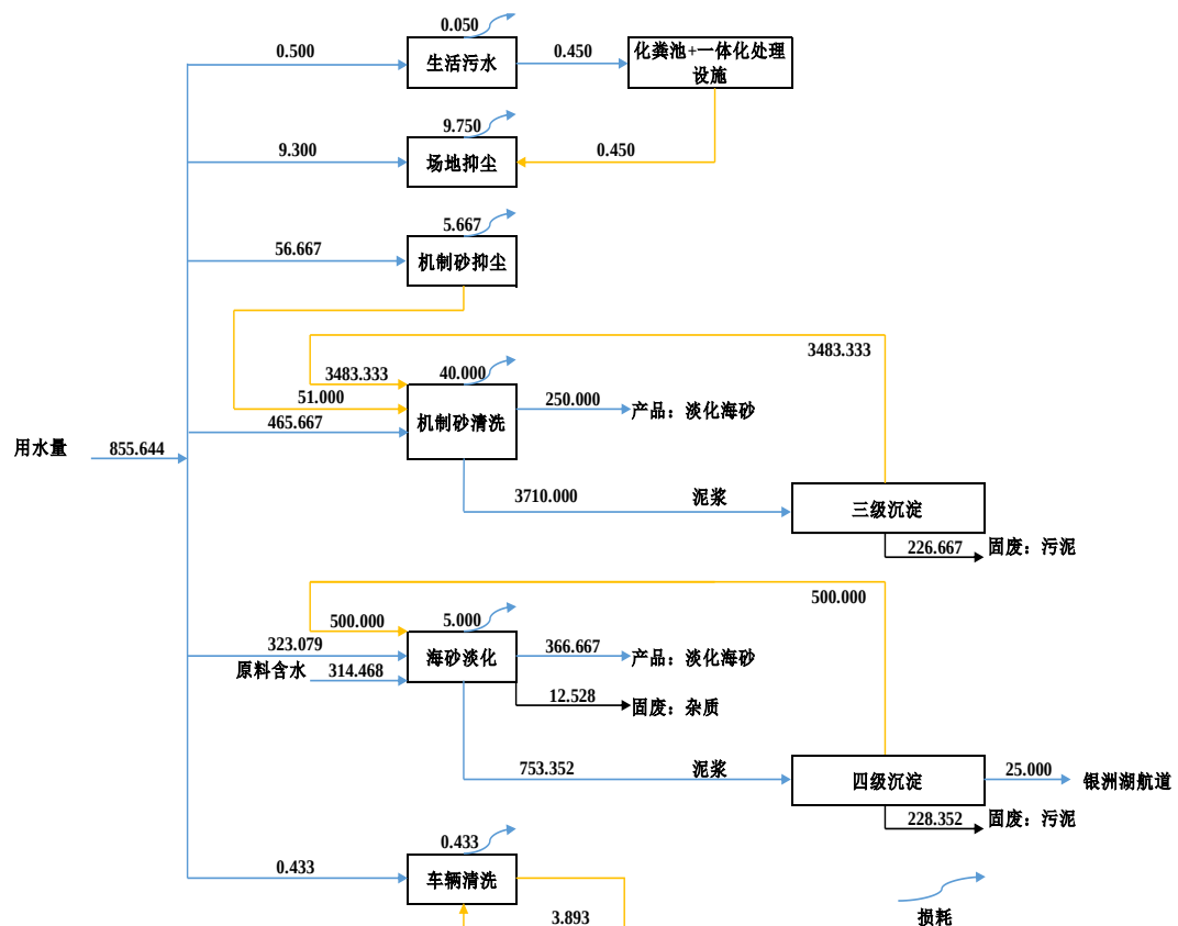
图1. 项目旱季水平衡图 (m 3 /d)
