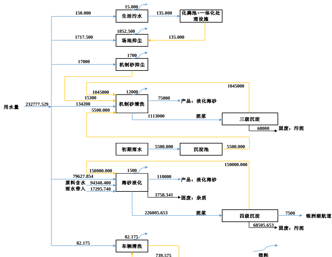
图3. 项目总水平衡图 ( \text{m}^3/\text{a} )
