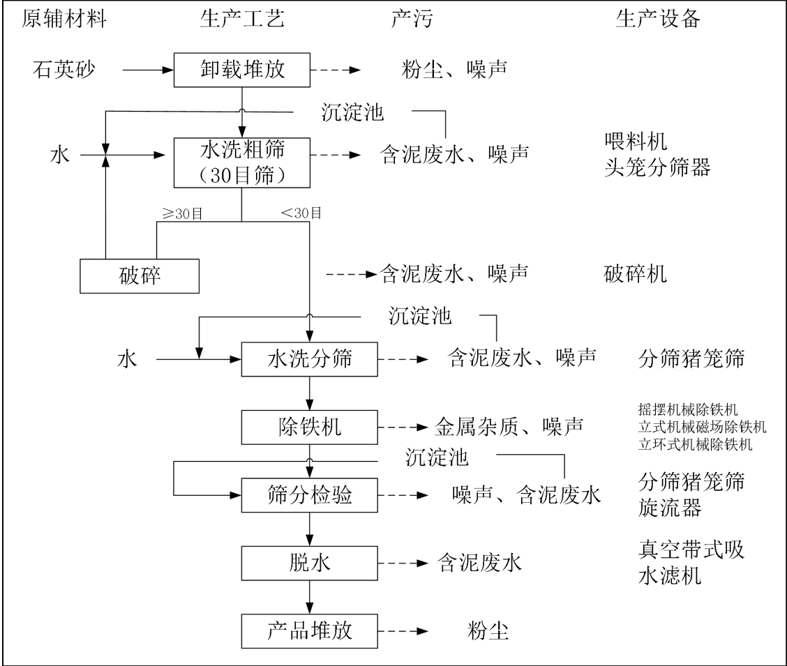
图 2-3 硅砂生产工艺流程图
