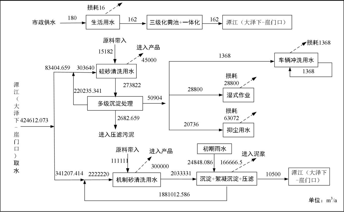
图 2-1 扩建项目水平衡图
