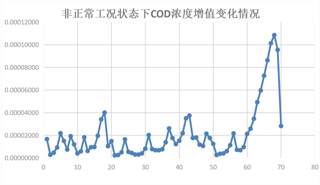
图 5.2-8 非正常排放情况排污口区域 COD Cr 浓度增值变化情况
