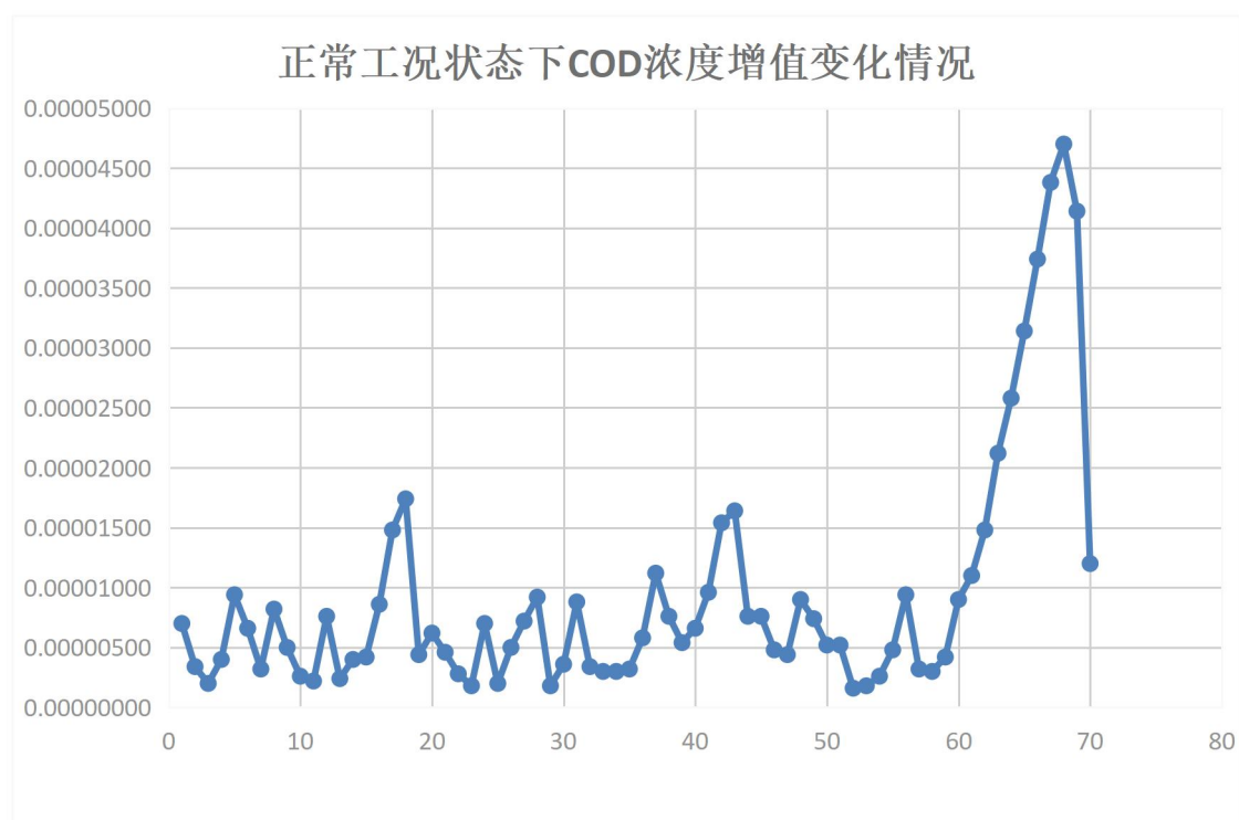
图 5.2-6 正常排放情况排污口区域 COD Cr 浓度增值变化情况
