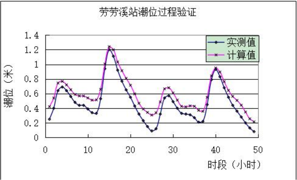
图 5.2-3 潭江（大泽下-崖门口）站 1999 年 7 月潮位验证图
