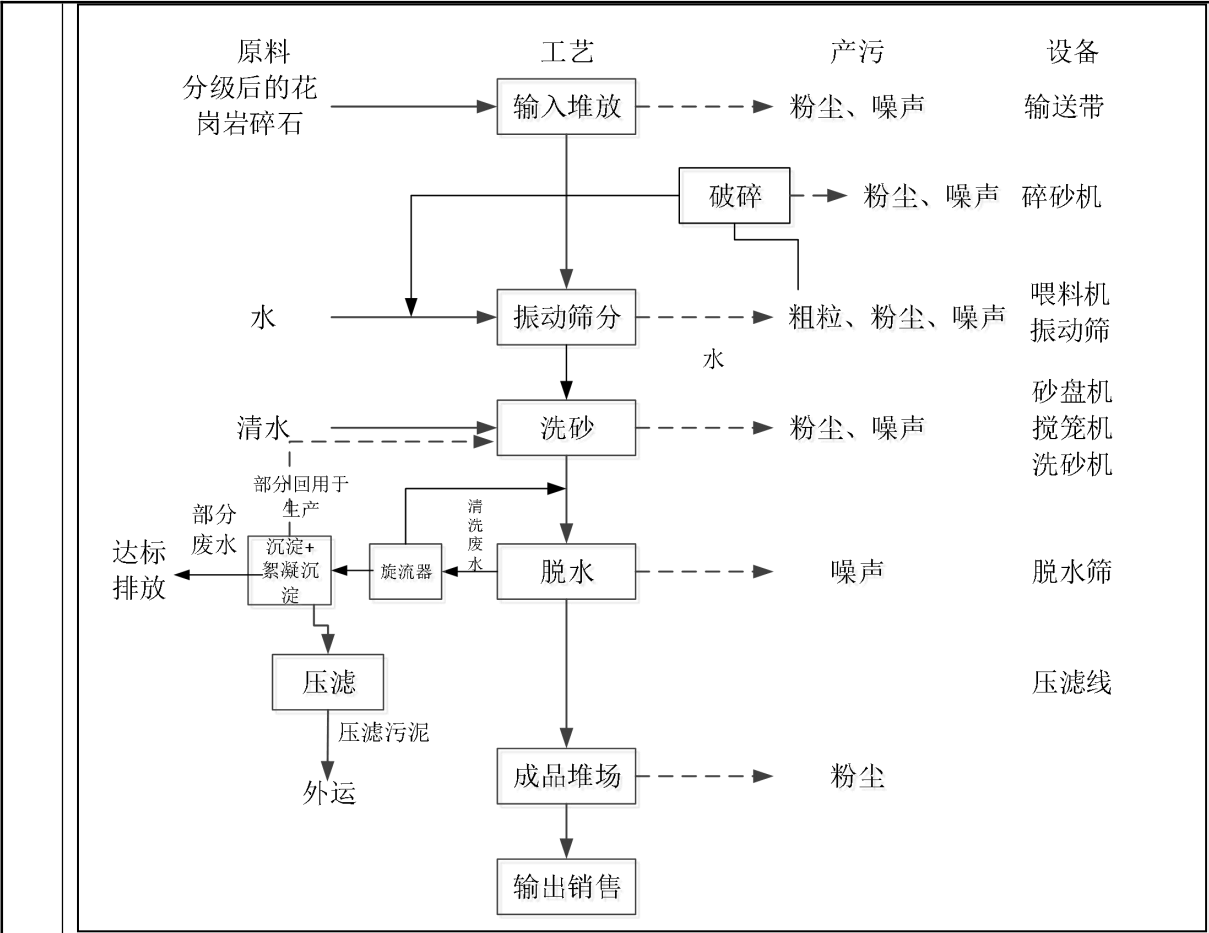
图 2-3 机制砂生产工艺流程图
