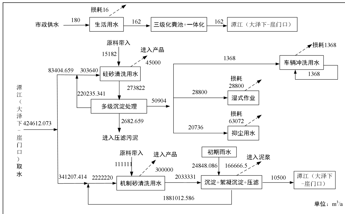
图 2.2-1 项目水平衡图
