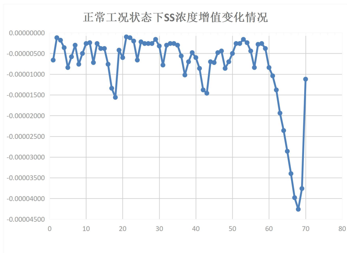
图 5.2-7 正常排放情况排污口区域 SS 浓度增值变化情况
