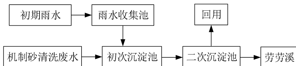
图 6.2-2 机制砂股废水处理工艺流程图
