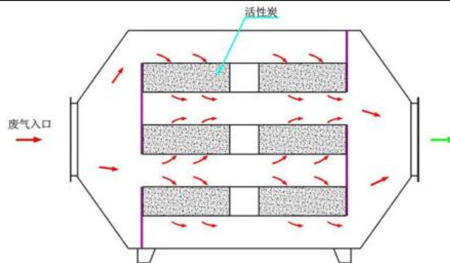
图 4-1 活性炭箱结构图
