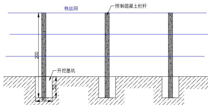
图 5-6 防护栏杆布置示意图
