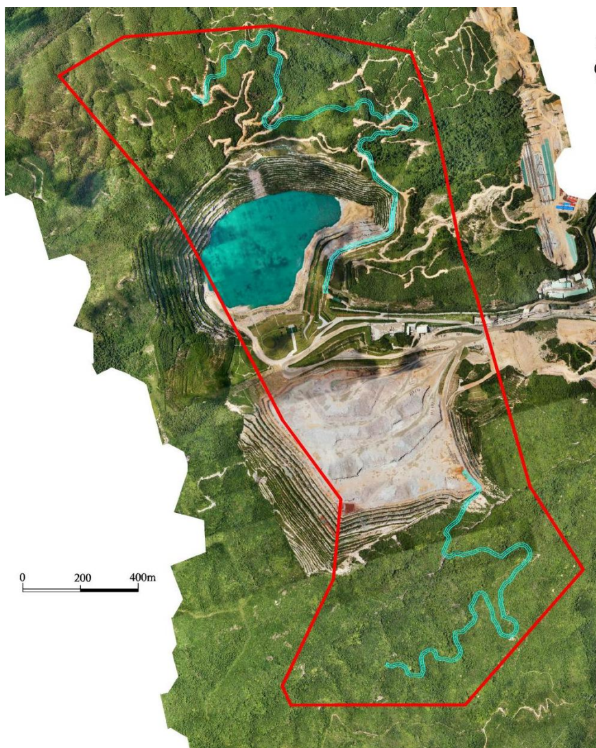
图 3-4 拟设矿山公路位置正射示意图（影像拍摄时间 2023 年 3 月）
