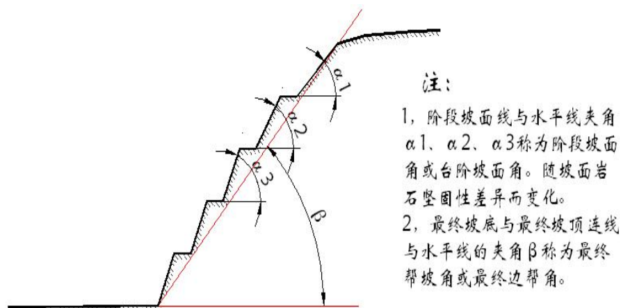
图 1-10 最终边坡构成要素图
