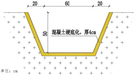
图 5-2 矿山公路内侧排水沟截面示意图
