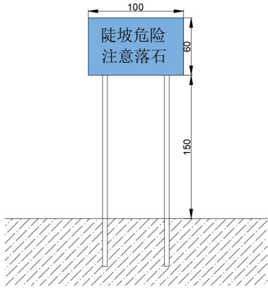
图 5-7 警示牌布置示意图
