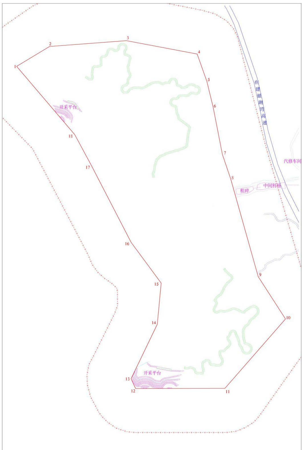
图 1-6 矿区基建终了平面图(一)(资料来源于开发利用方案)
