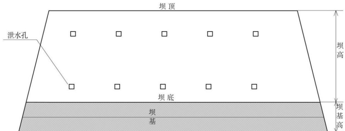
图 5-4 拦渣坝横截面示意图
