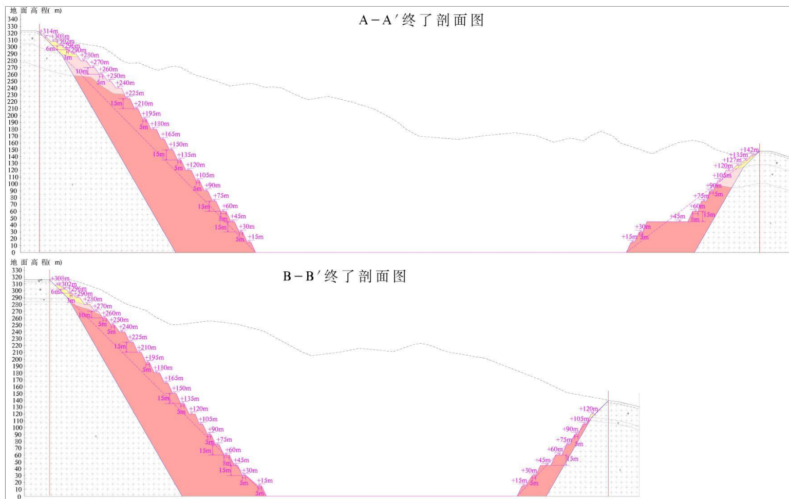
图 1-9 矿区开采剖面图(资料来源于开发利用方案)
