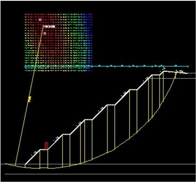
[计算结果图]
