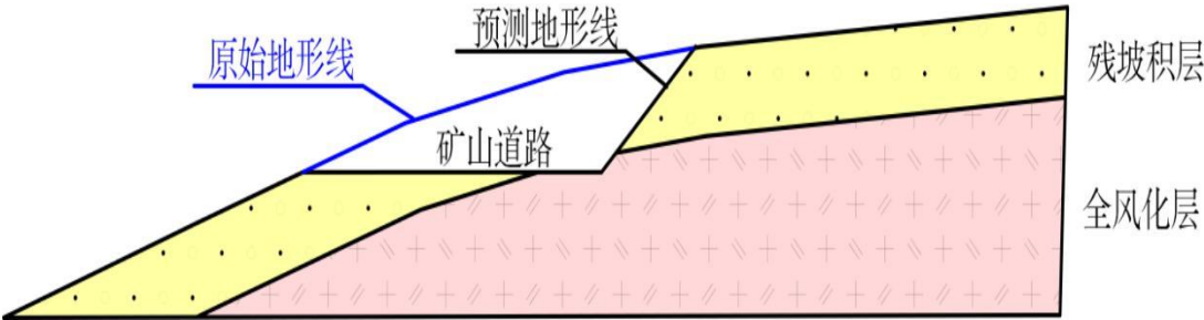
图 3-3 山坡露天开采时矿山公路边坡剖面示意图
