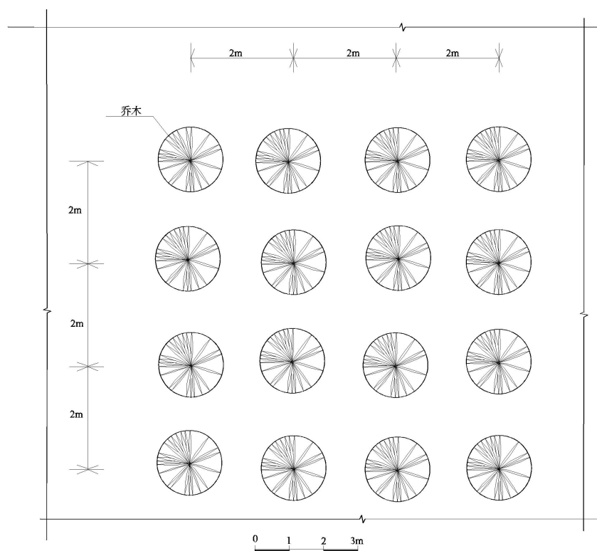
图 5-12 办公生活区绿化示意图
