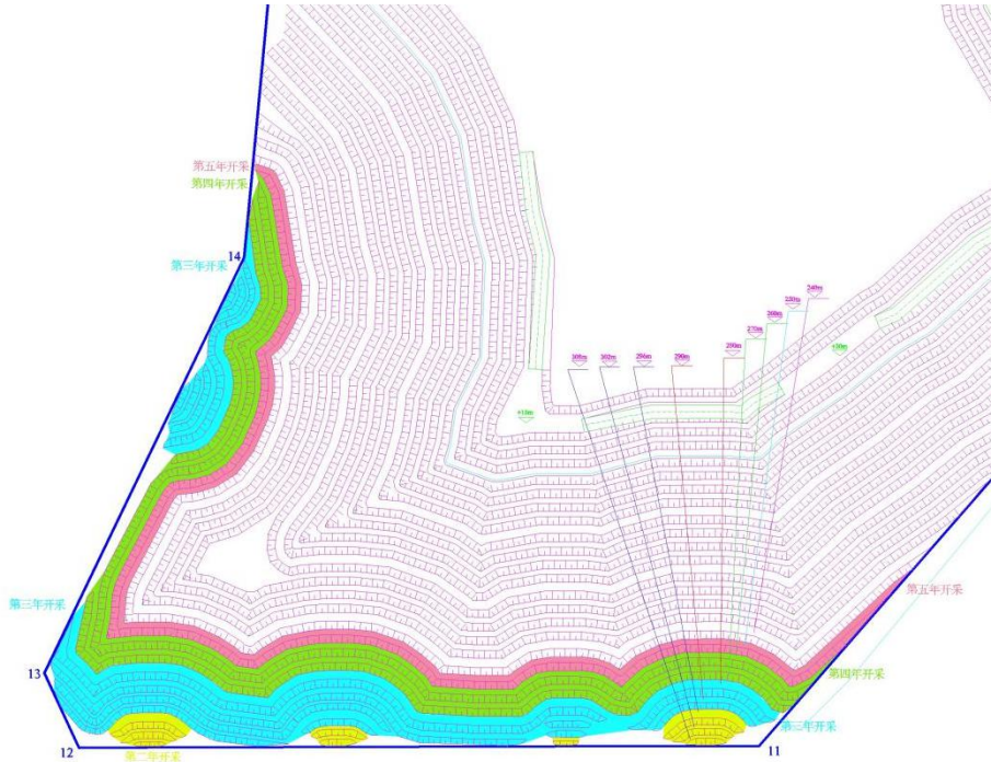
图 6-1 近期开采形成边坡台阶示意图
