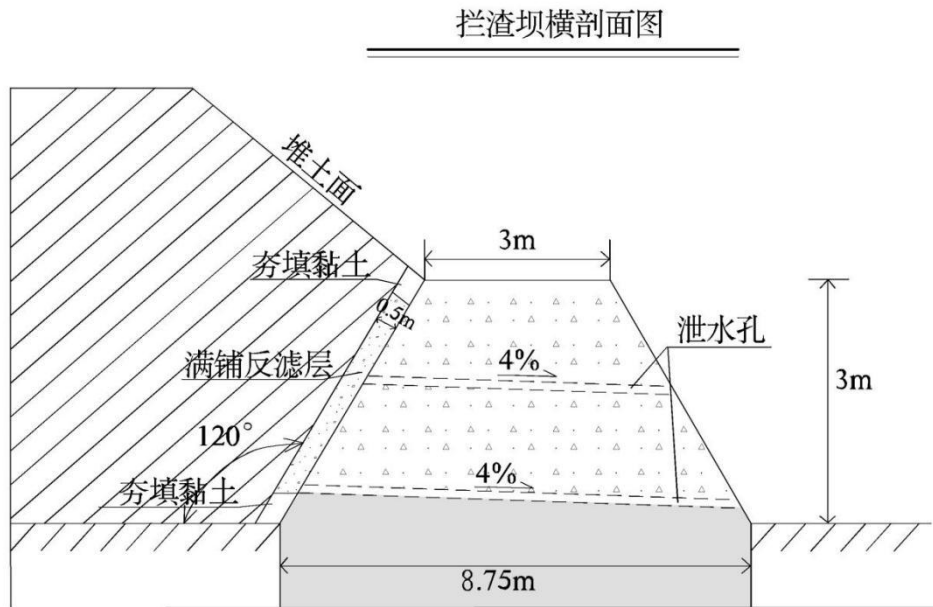
图 5-3 拦渣坝横截面示意图
