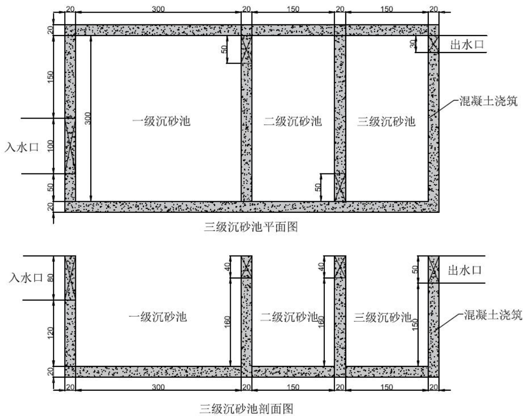
图 5-16 沉砂池工程大样图
