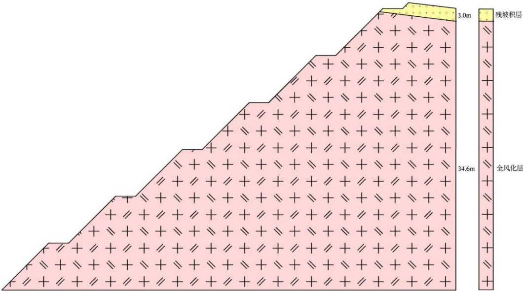
图 3-2 北部土质边坡结构示意图
