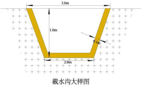
图 5-1 外围截排水沟设计规格
