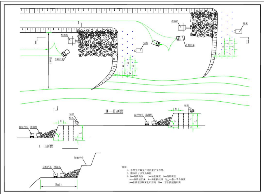
图 3-5 矿山露天开采工艺示意图
