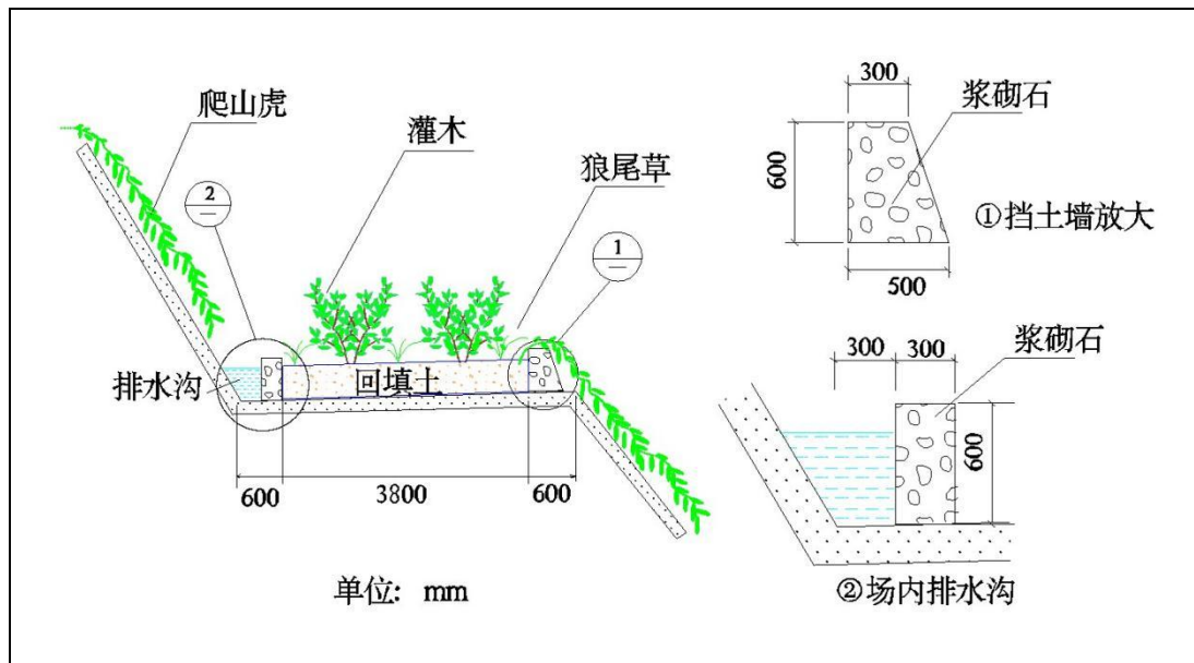
图 5-7 露天采场台阶植被设计规格
