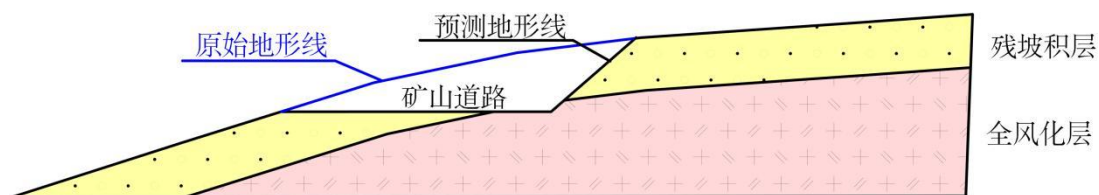
图 3-3 山坡露天开采时矿山公路边坡剖面示意图
