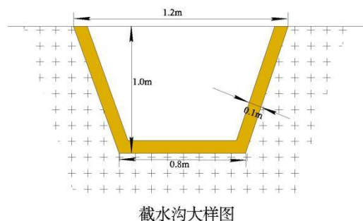
图 5-1 外围截水沟设计规格
