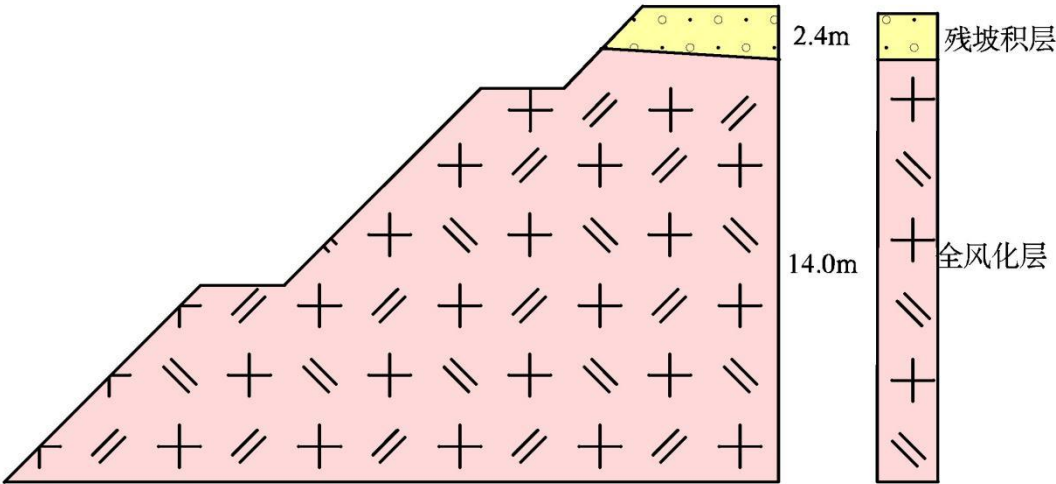
图 3-2 北部土质边坡结构示意图
