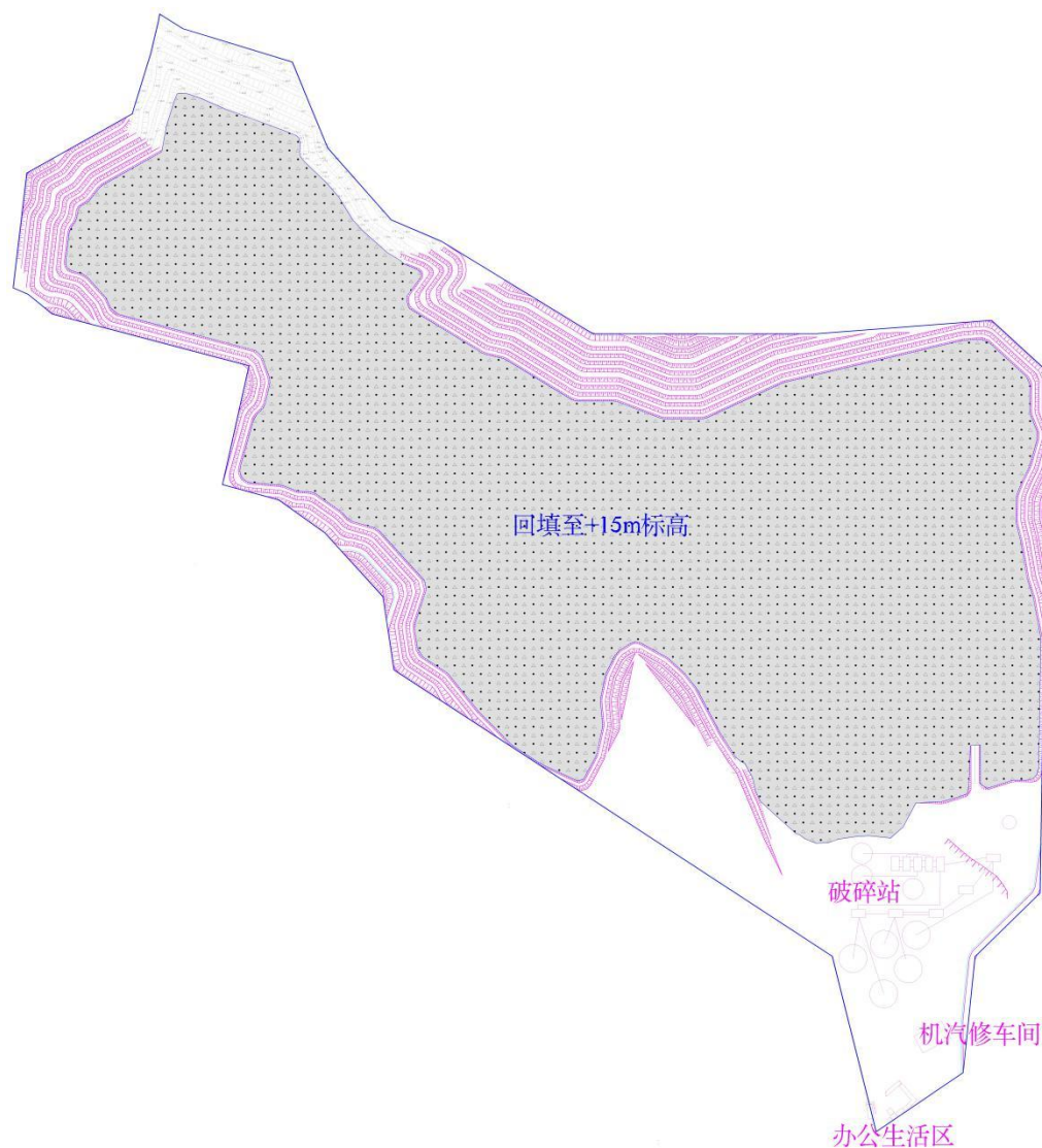
图 4-1 露天采场终了场内平整示意图
