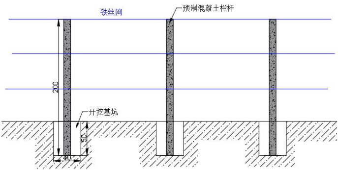
图 5-3 防护栏杆布置示意图
