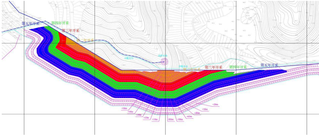
图 6-1 近期开采形成边坡台阶示意图
