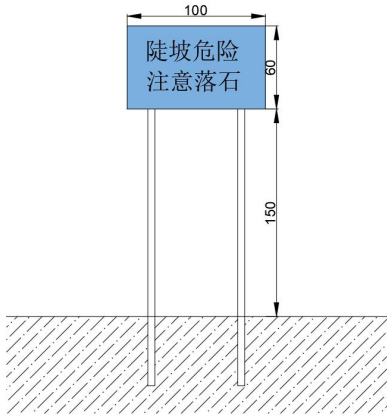
图 5-4 警示牌布置示意图
