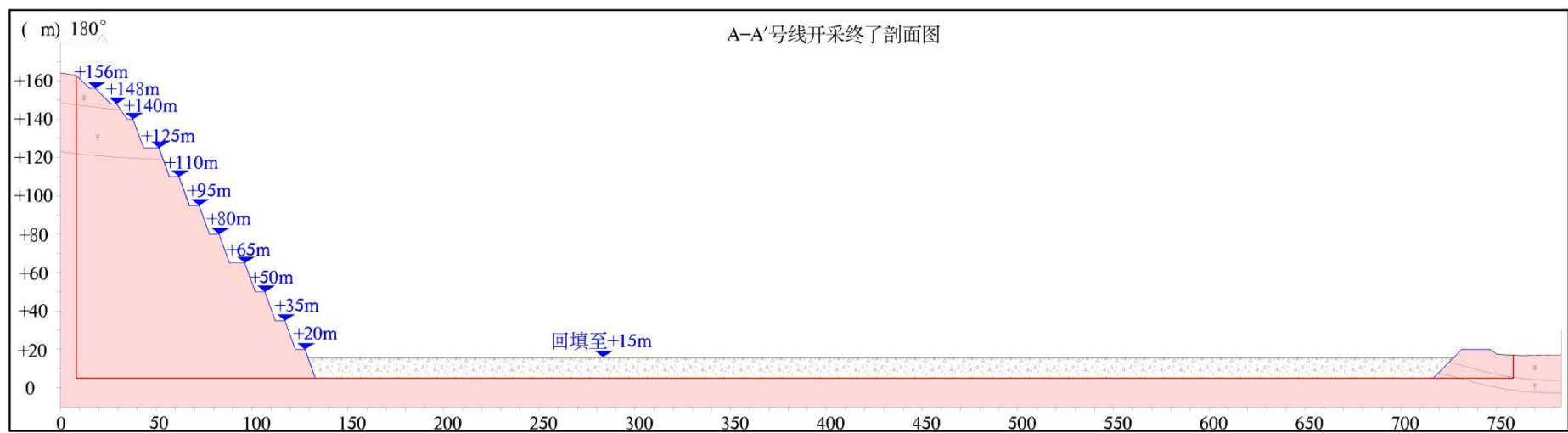
图 1-7 矿区开采剖面示意图(资料来源于开发利用方案)
