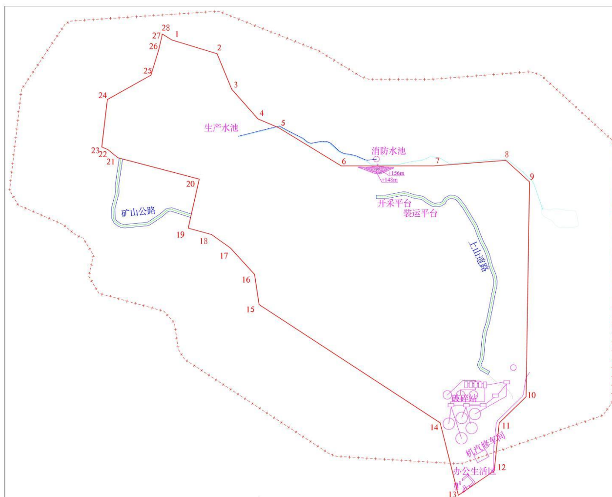
图 1-5 矿区基建终了平面示意图(资料来源于开发利用方案)
