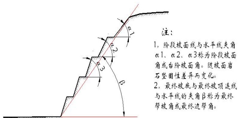
图 1-8 最终边坡构成要素图
