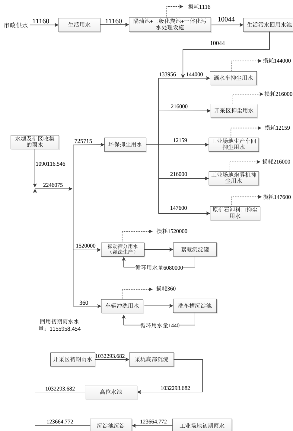
图 2-8 项目水平衡示意图 (单位: m 3 /a)
