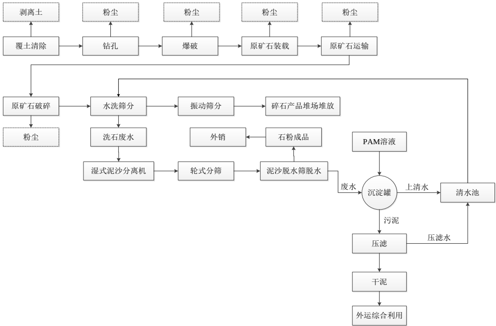
图 2-4 项目生产工艺流程图
