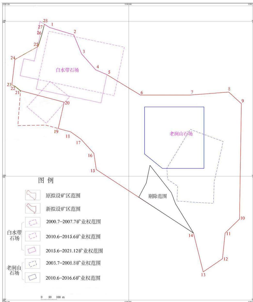
图 2-1 矿区采矿权位置图
