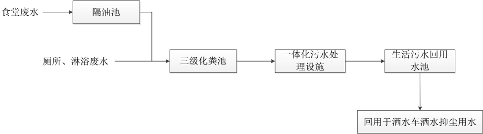
图 4-2 生活污水处理工艺流程图
