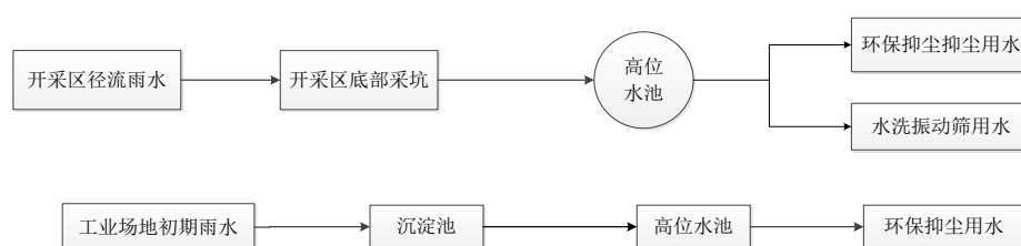
图 5-3 项目初期雨水处理工艺流程图
