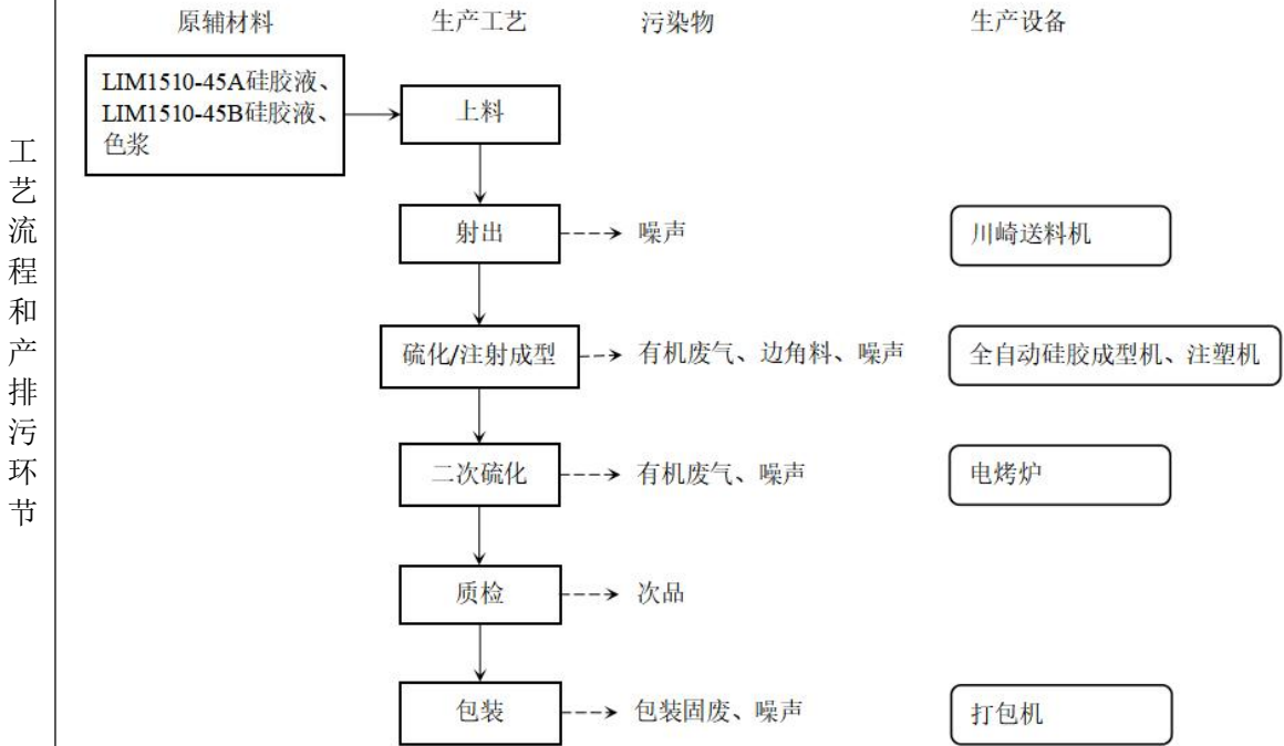
图2-2 硅胶制品生产工艺流程图
