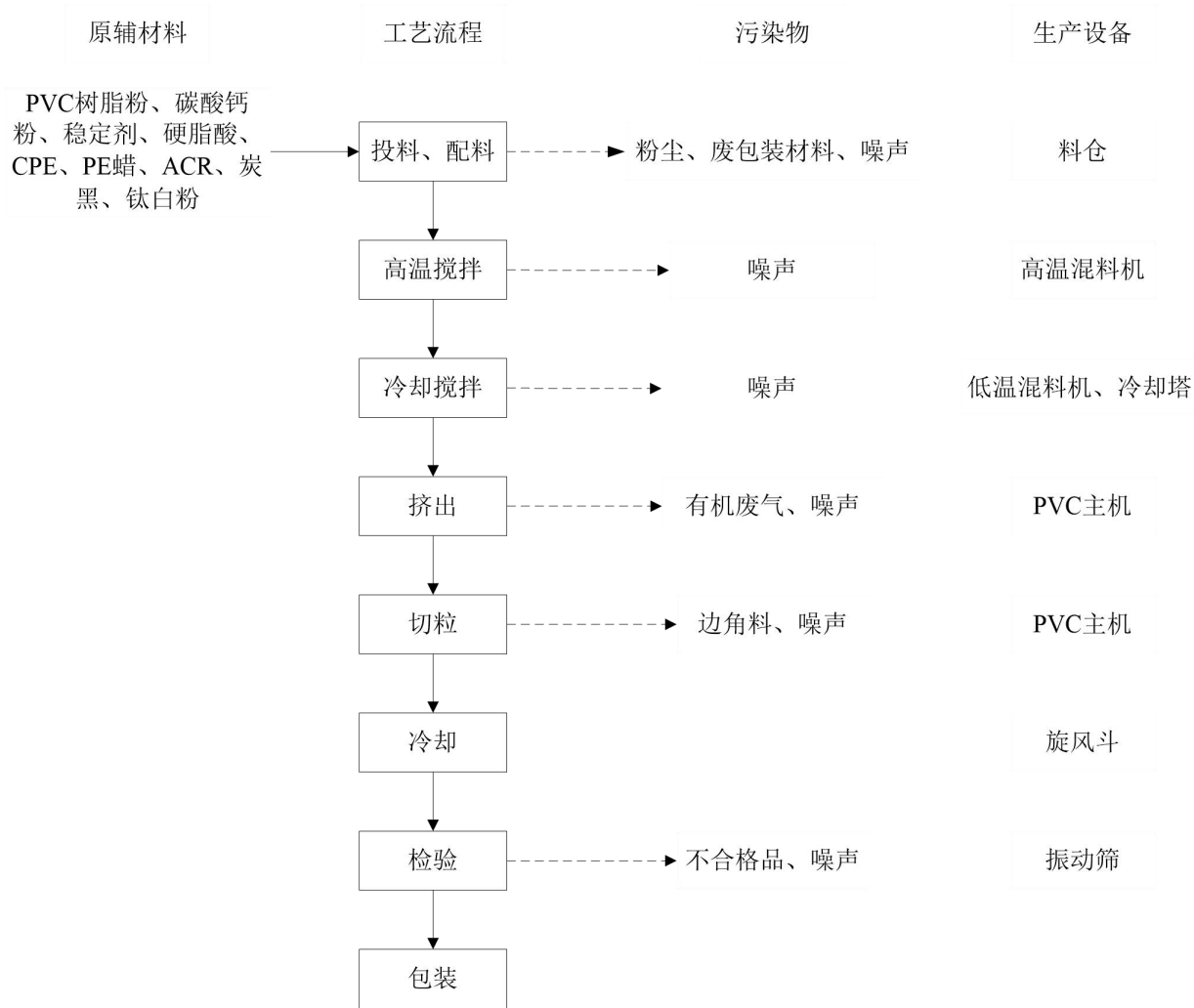
图 2-2 改性塑料粒生产工艺流程及产污环节图
