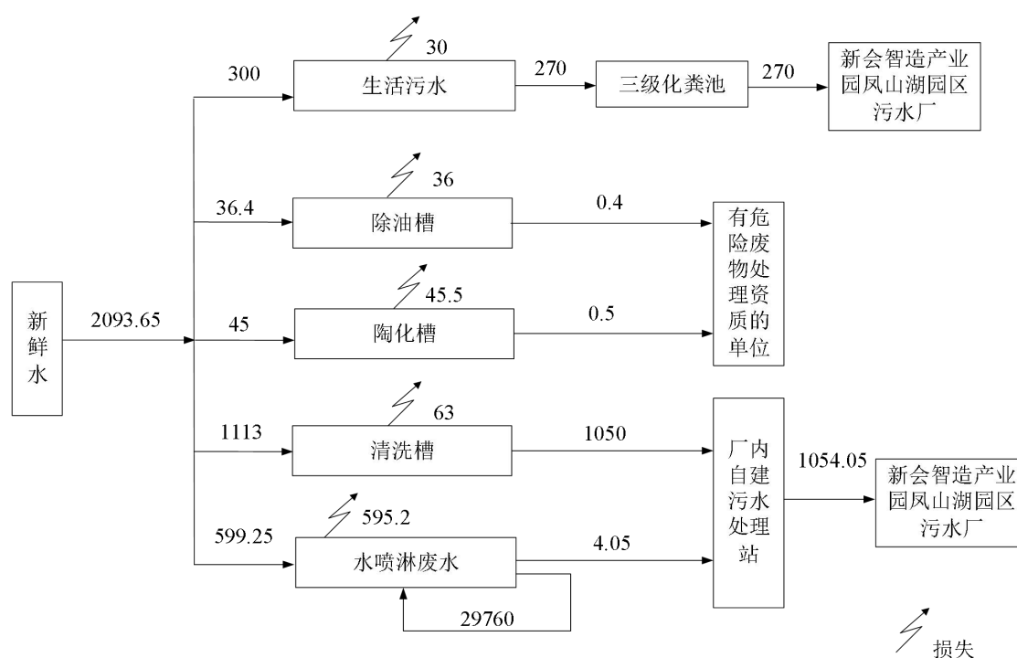
图 1. 项目水平衡图 (t/a)
