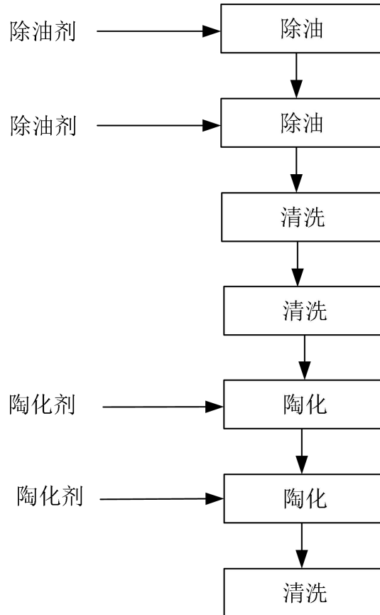
图 2. 前处理线生产工艺流程图
