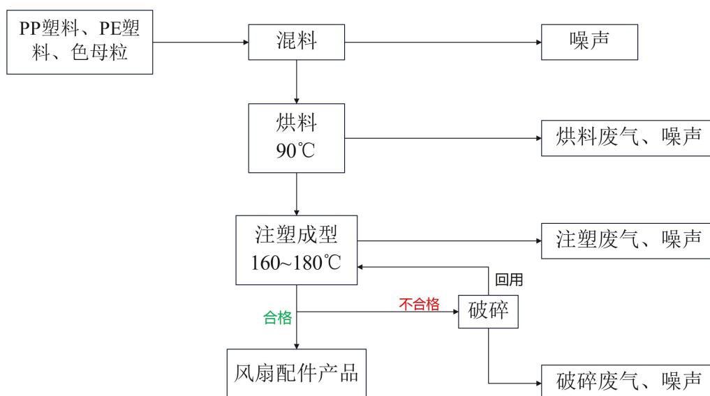
风扇配件生产工艺流程图
