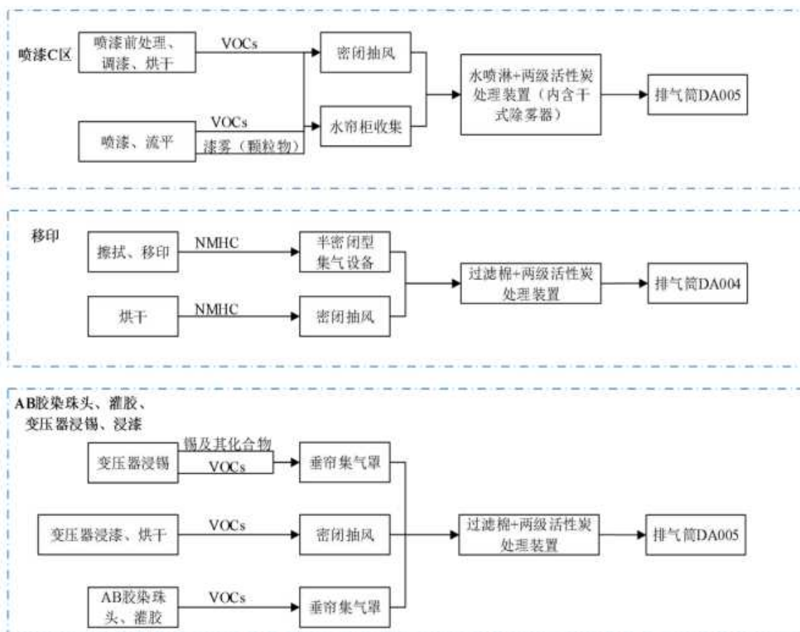
图5.1-1有组织废气治理收集走向示意图（二）
