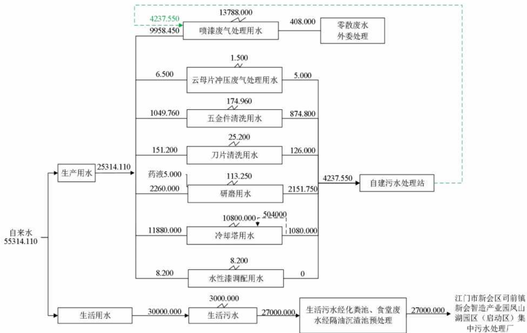
图2.3-3建设项目水平衡图 (单位: \text{m}^3/\text{a} )
