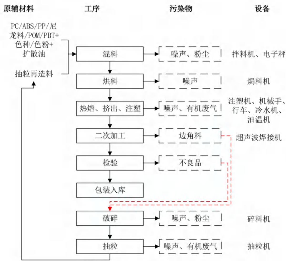
图2.2-5注塑生产工艺流程及产污节点图
