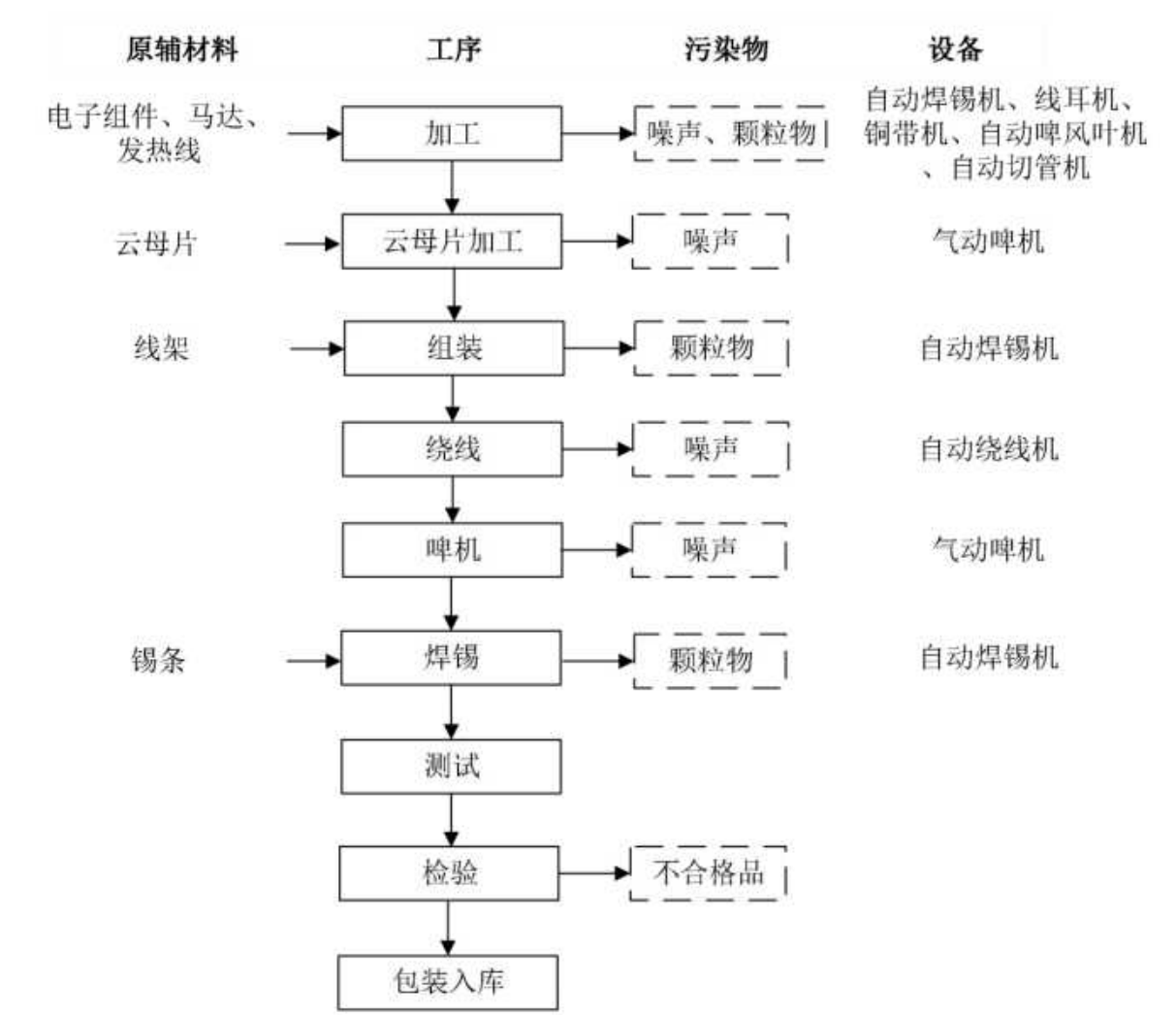
图2.2-10线架生产工艺生产流程及产污节点图
