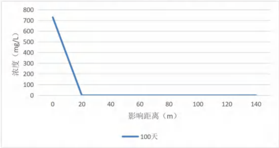
图4.4-1COD污染物连续渗漏100d情况预测统计图
