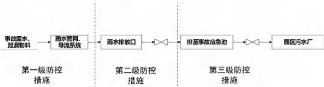
图4.9-1三级防控体系示意图
