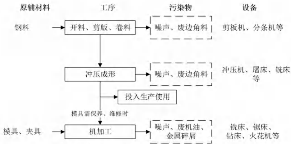
图2.2-1模具及夹具制作及维修流程及产污节点图
