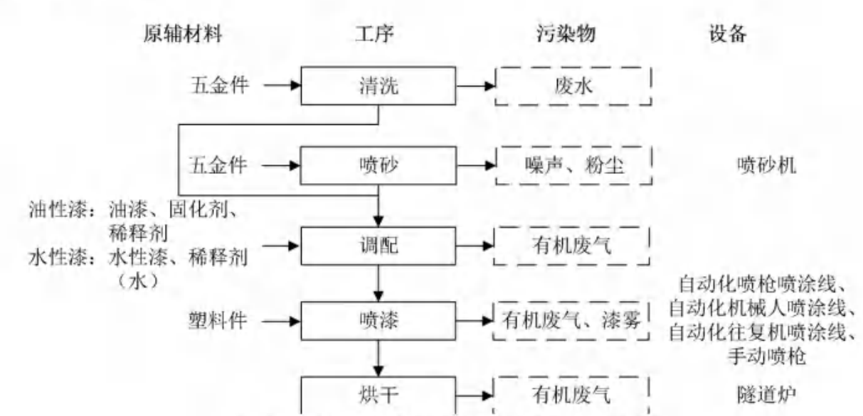
图2.2-6喷漆工艺生产流程及产污节点图
