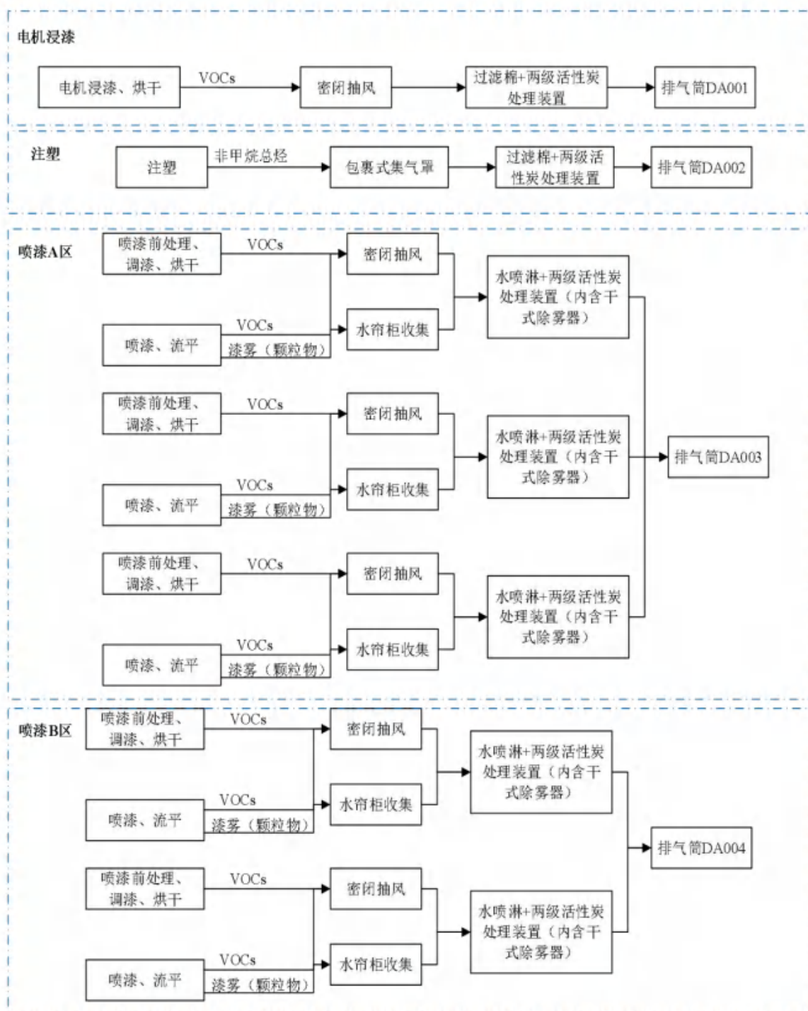
图5.1-1有组织废气治理收集走向示意图（一）
