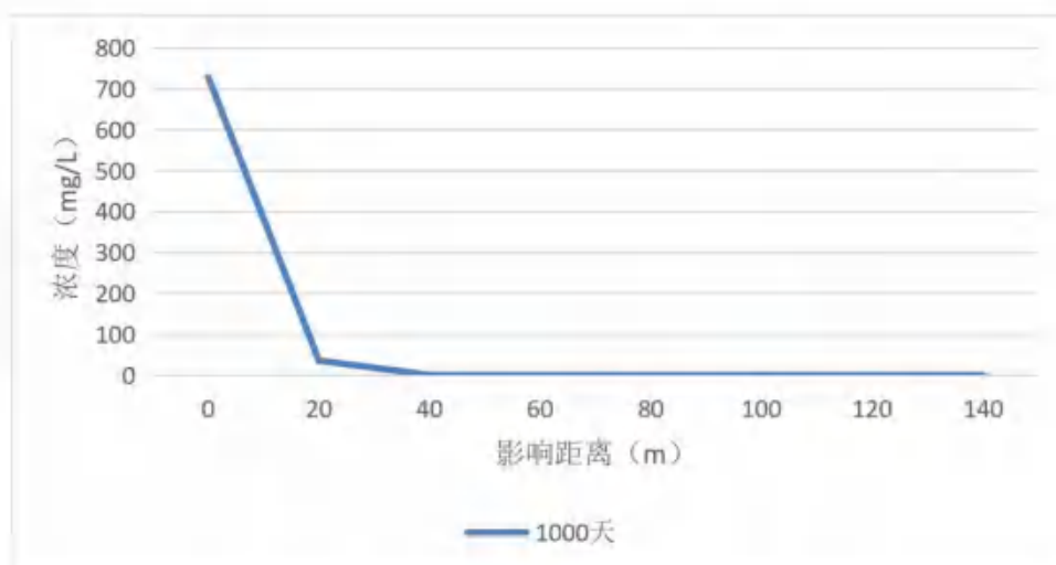
图4.4-2COD污染物连续渗漏1000d情况预测统计图
