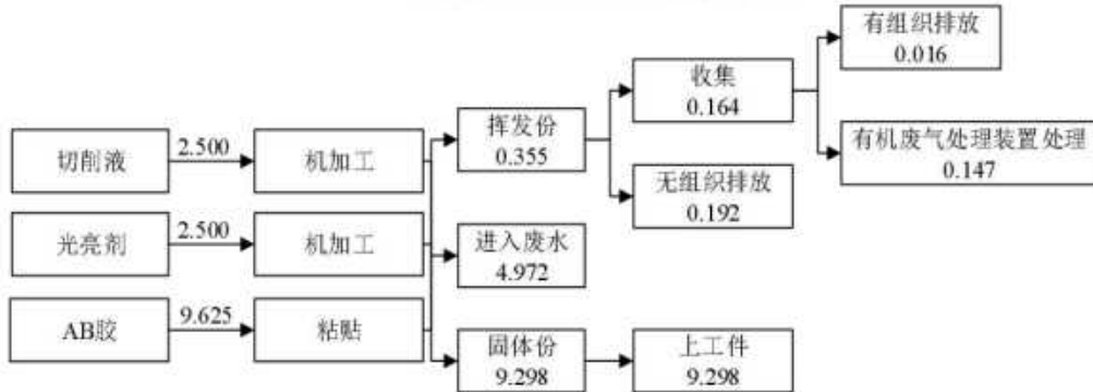
机加工过程VOCs物料平衡
