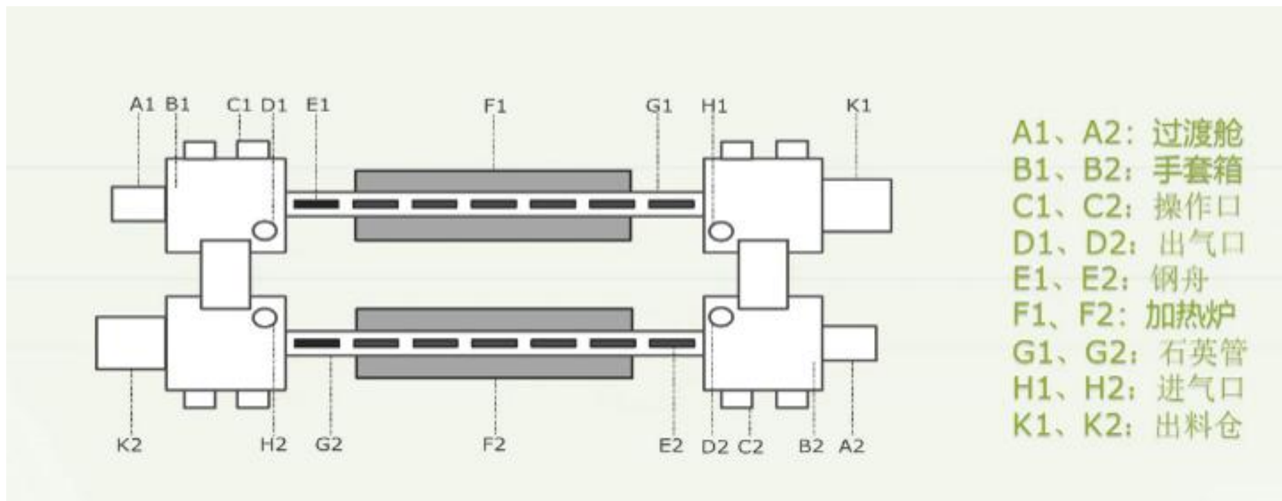
图 3.2-5 粗管径碳纳米管的生产设备连接图
