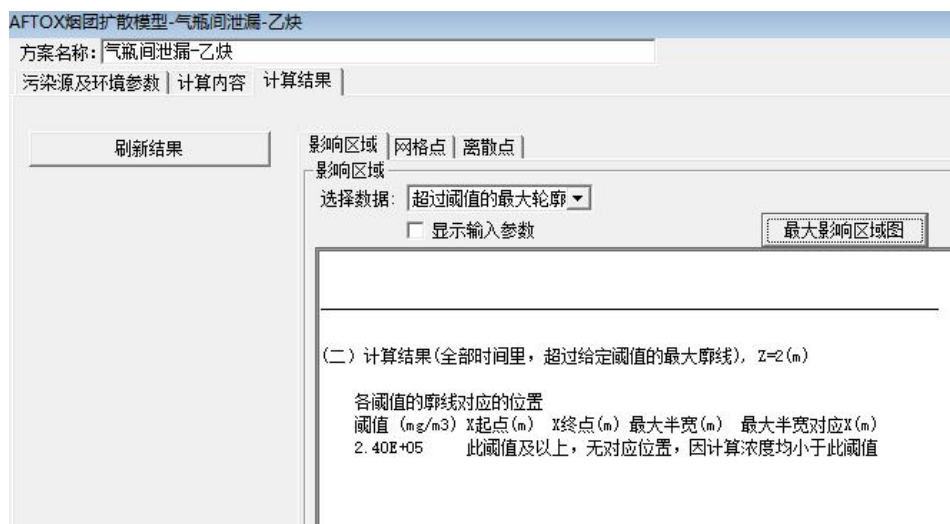
图6.6-3 下风向不同距离处气瓶间泄漏乙炔的超过阈值最大轮廓图
