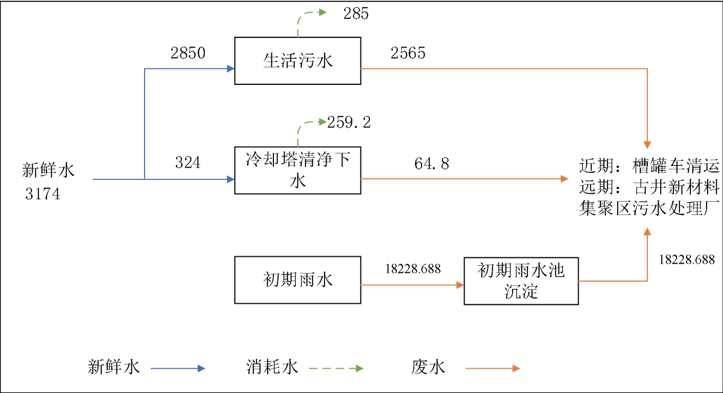
图 3.3-1 已批已建已验项目水平衡图 单位：m³/a
