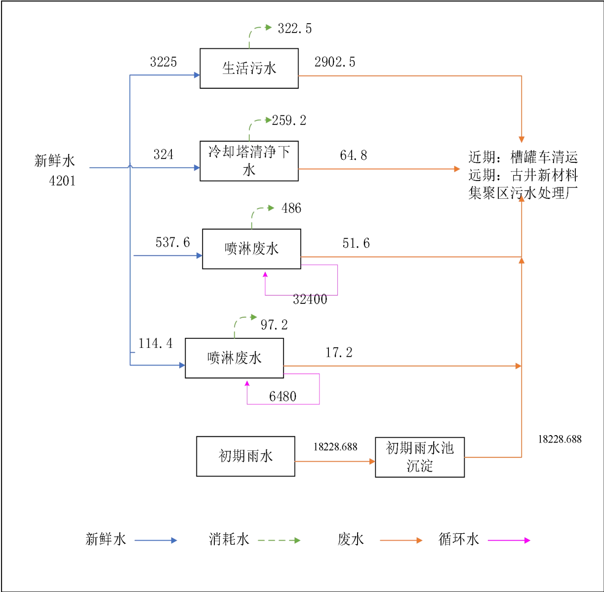
图 4.4-2 扩建后总体项目水平衡图 单位: m³/a
