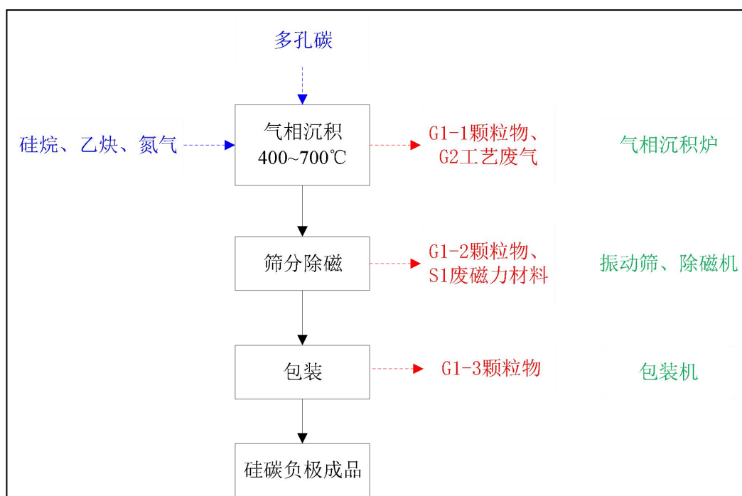
图 4.2-1 硅碳负极工艺流程
