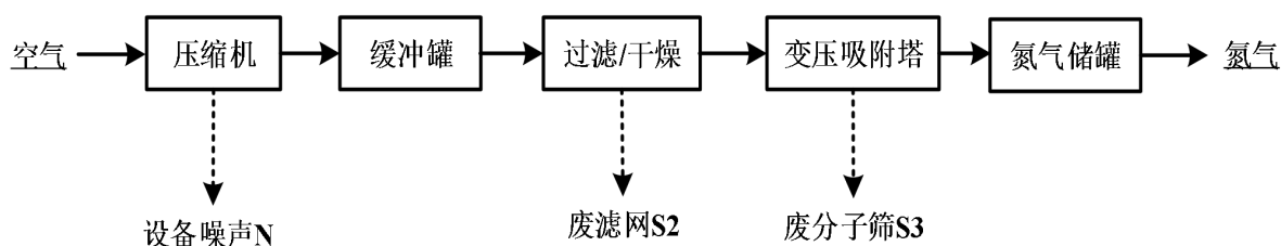
图 4.2-2 氮气制备工艺流程及产污环节
