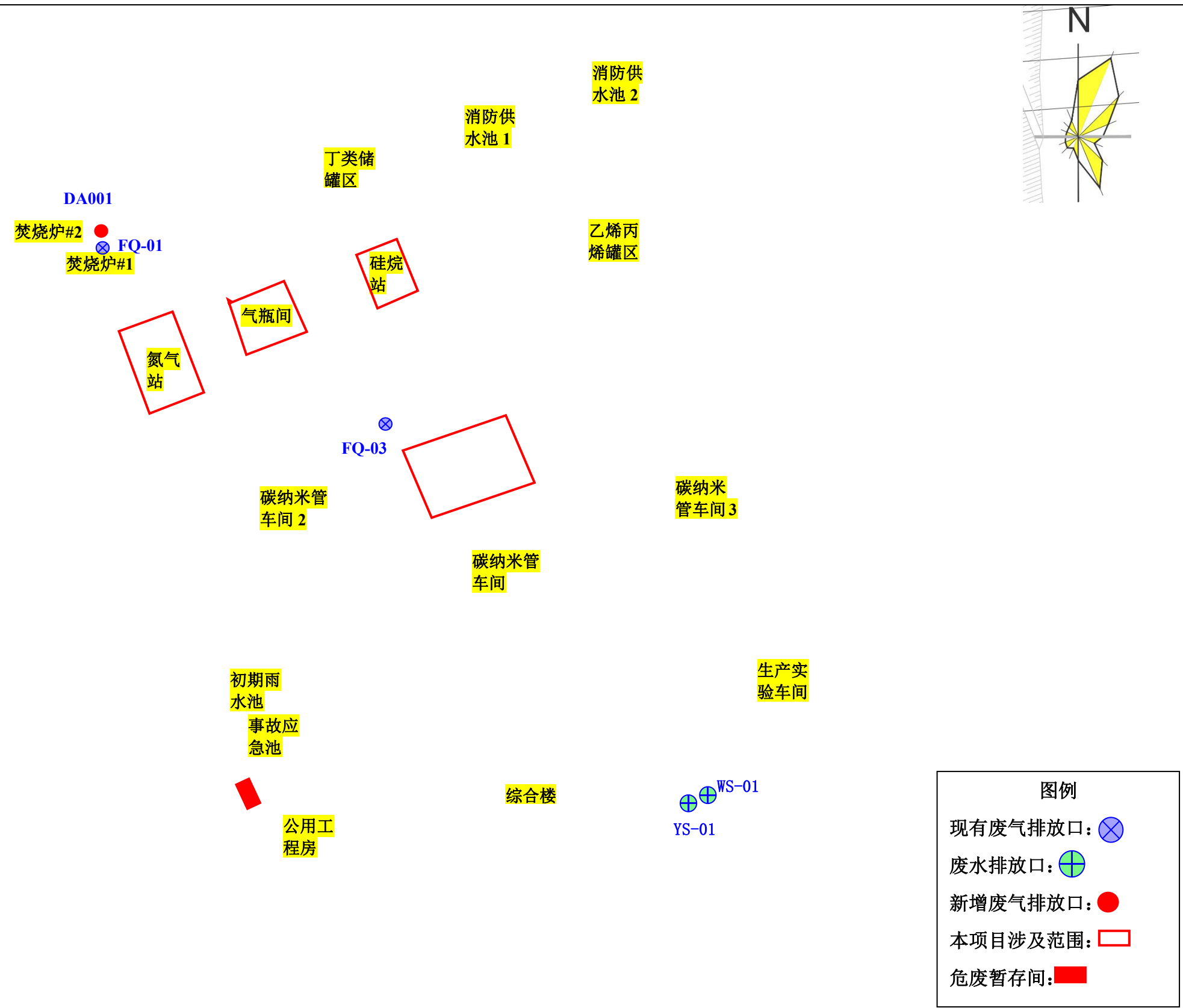
图 4.1-2 扩建后，总体项目总平面布置图
