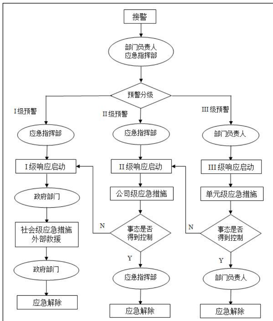
图 6.6-12 突发环境事件应急回应程序
