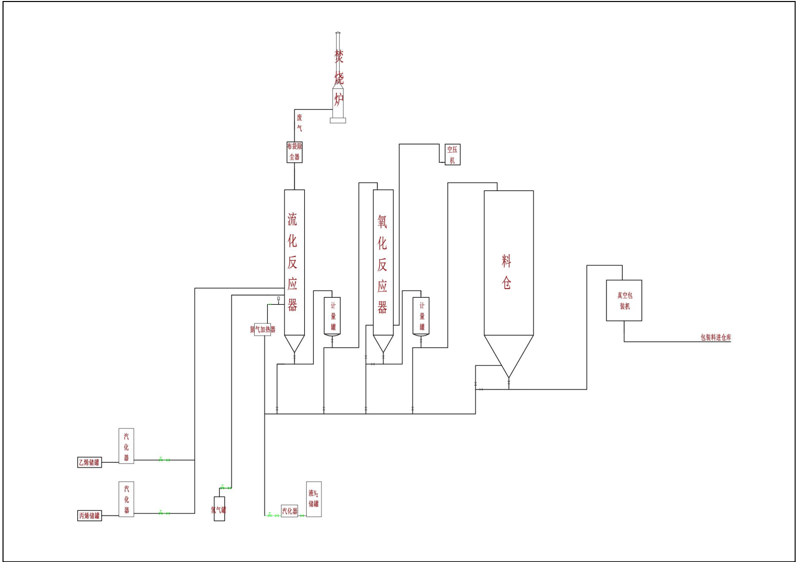
图 3.2-3 细管径碳纳米管的生产设备连接图
