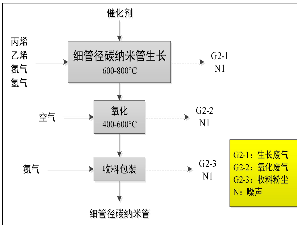
图3.2-2 细管径碳纳米管生产工艺流程图与产污环节
