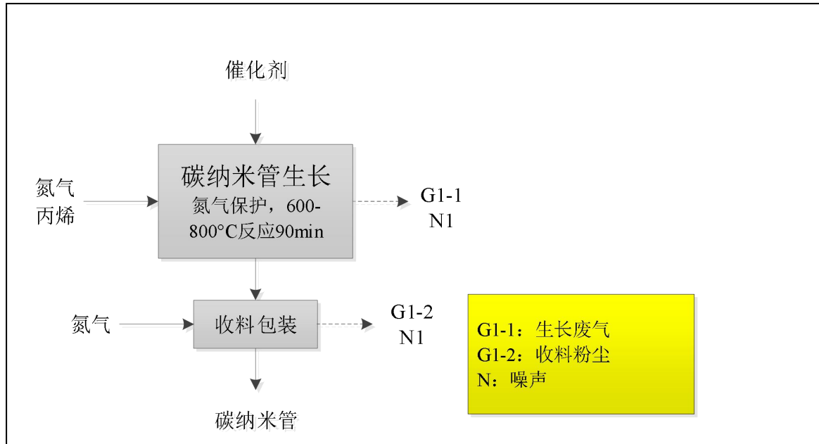
图3.2-1 碳纳米管生产工艺流程图与产污环节
