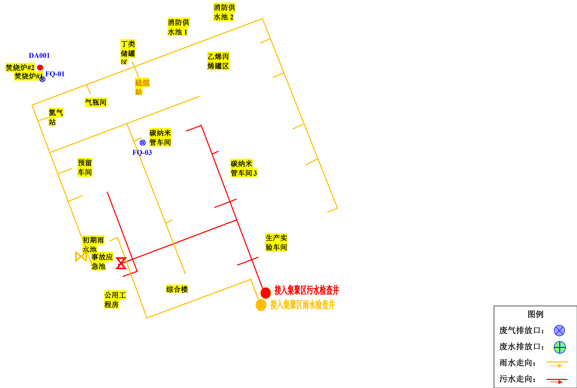
图 6.6-8 扩建后总体项目雨污管网图
