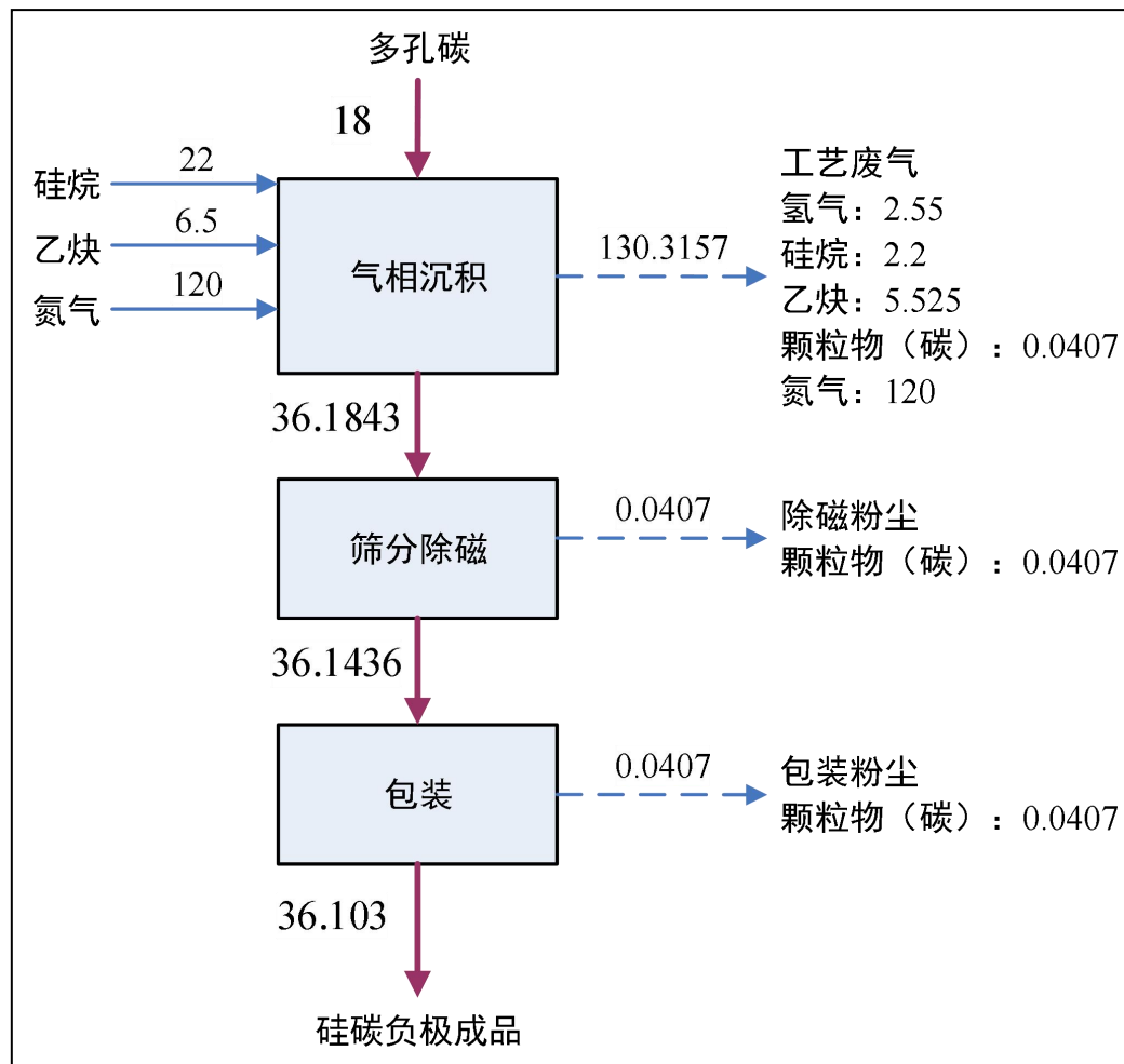
图 4.2-10 硅碳负极生产线物料平衡图（单位：t/a）
