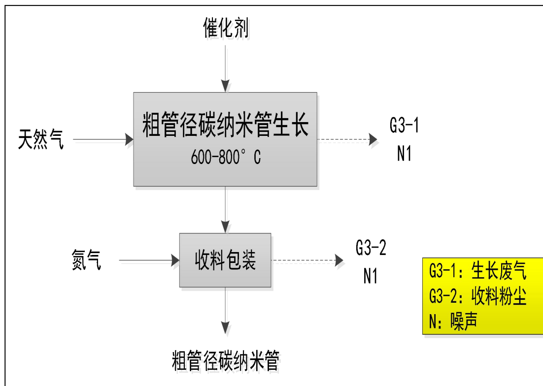
图 3.2-4 粗管径碳纳米管生产工艺流程图与产污环节
