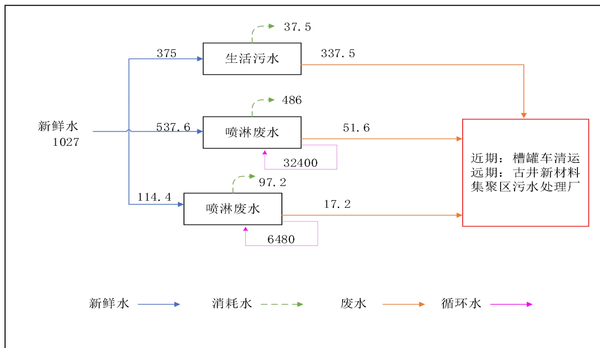
图 4.4-1 扩建项目水平衡图 单位：m 3 /a
