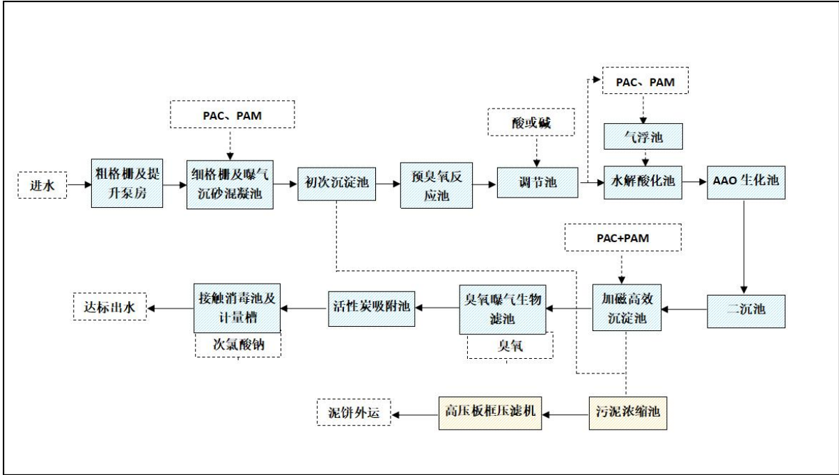
图 6.1-1 污水处理站工艺流程图
