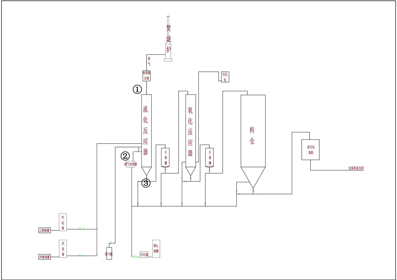
图 3.3-3 现有项目废气收集设施示意图
