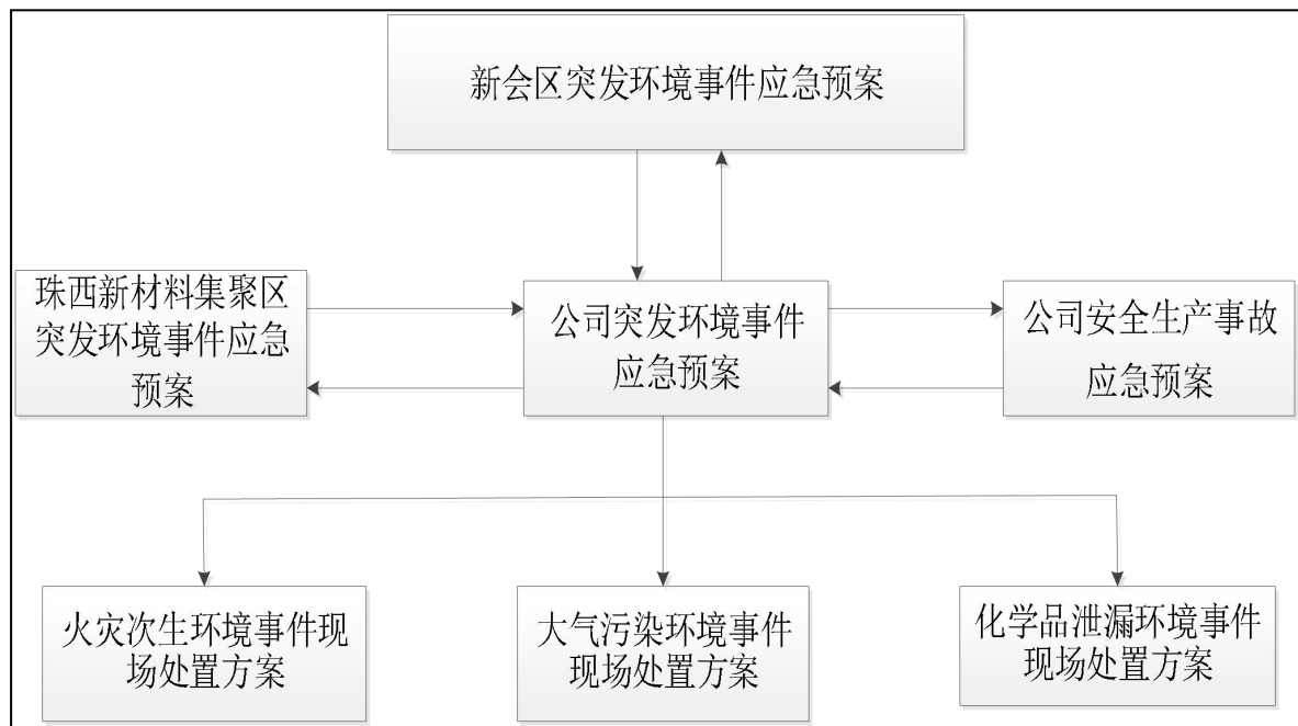
图 6.6-9 各应急预案关系图
