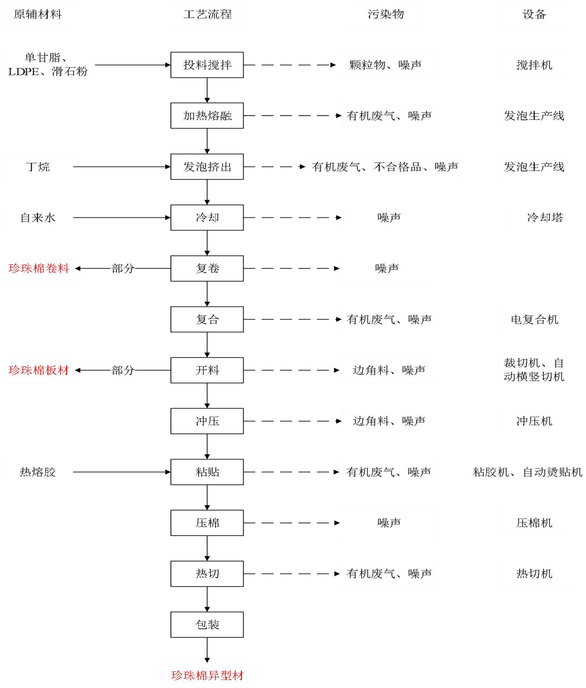
图 2-2 珍珠棉生产工艺流程及产污环节图
