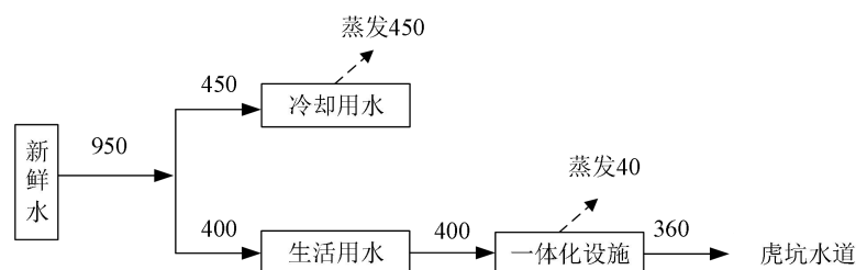
图 2-1 近期项目水平衡图（单位： \text{m}^3/\text{a} ）
