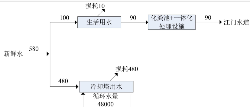
图 1. 项目水平衡图（近期）（t/a）
