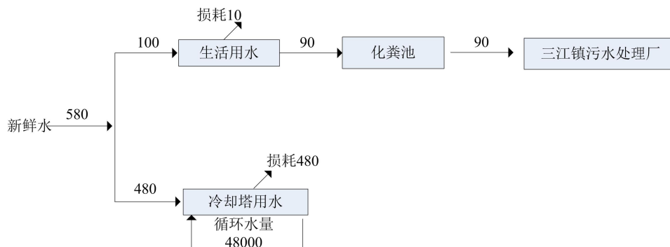
图 2. 项目水平衡图（远期）（t/a）
