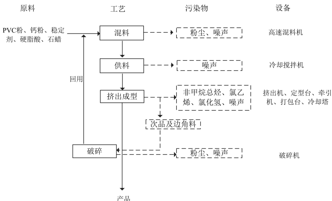
图 3. 塑料配件生产工艺流程及产污环节
