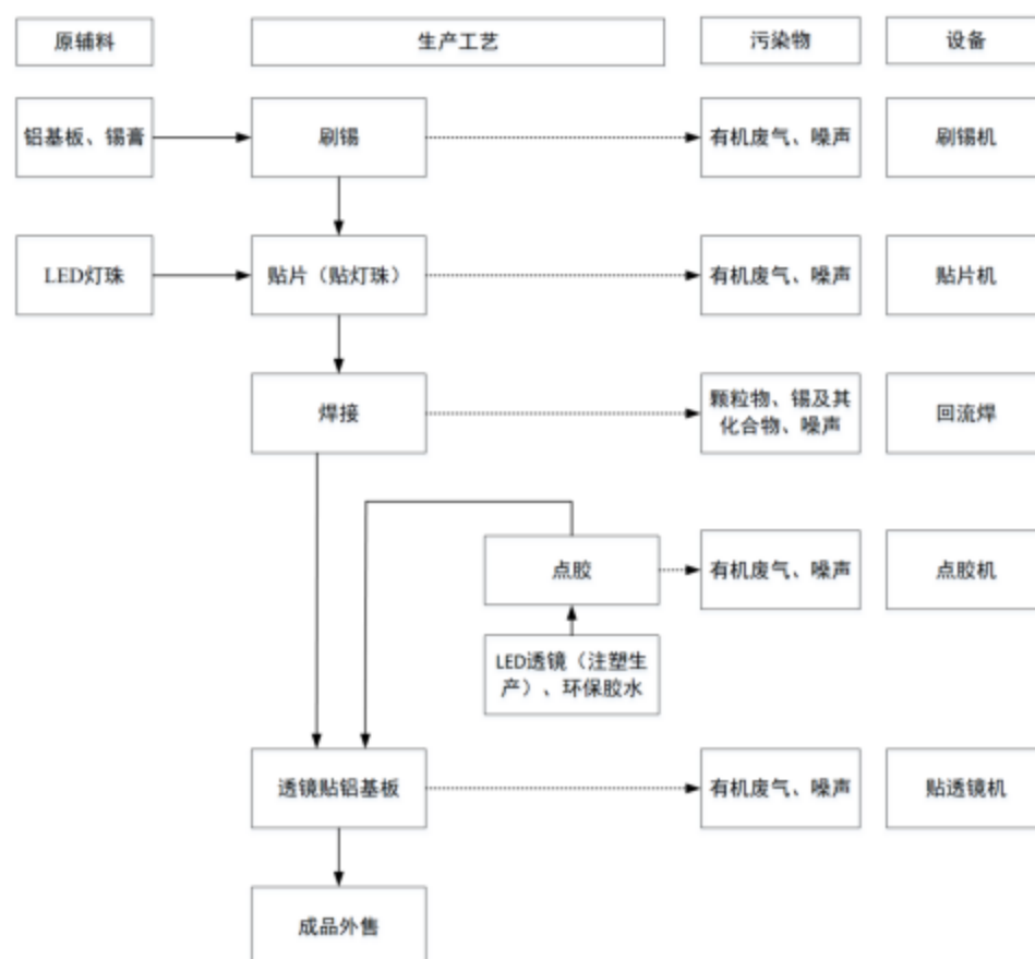
图 2-2 LED 透镜生产工艺流程图
