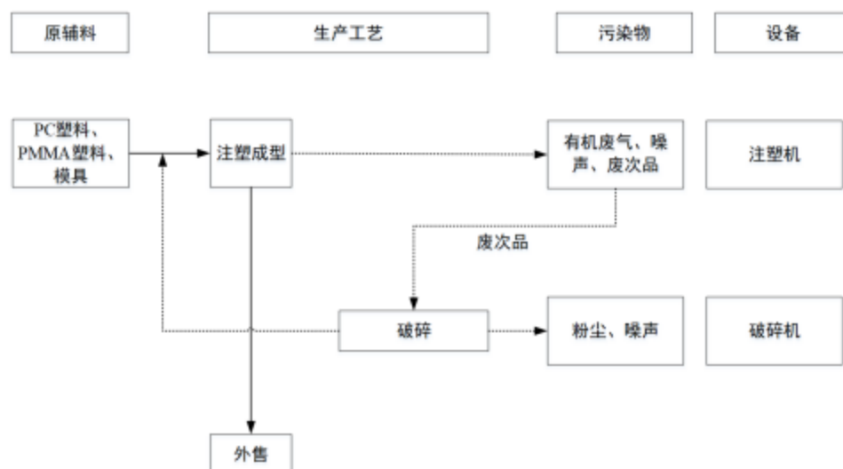
图 2-2 LED 透镜生产工艺流程图
