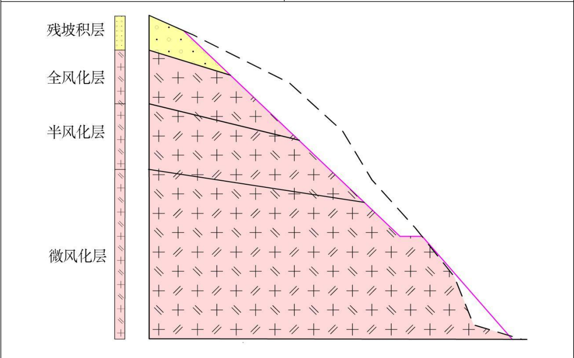
图 3-9 边坡结构示意图
