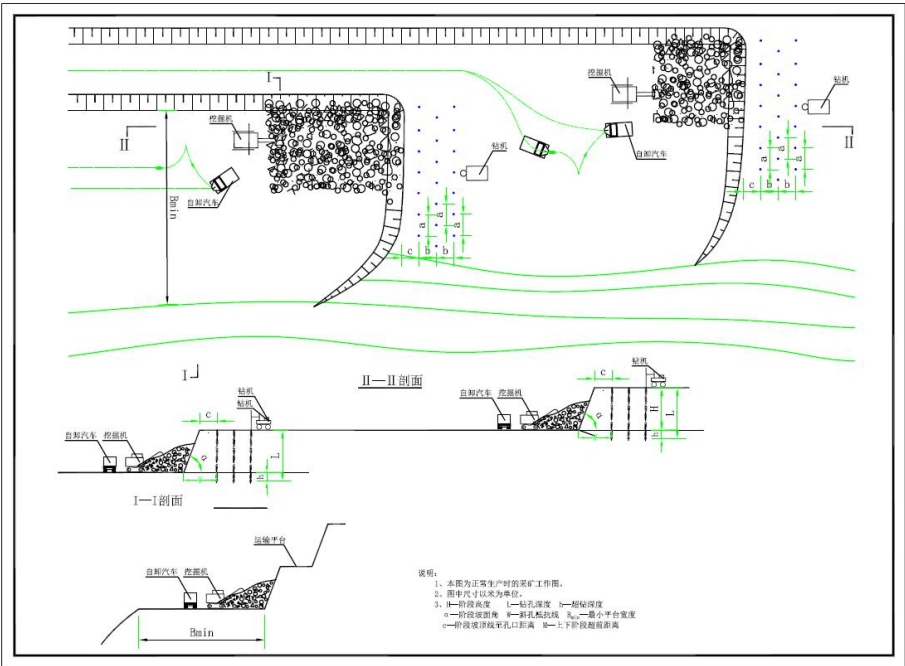
图 3-10 矿山露天开采工艺示意图
