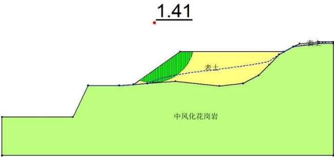
自然工况 Morgenstern-Price 法计算结果
