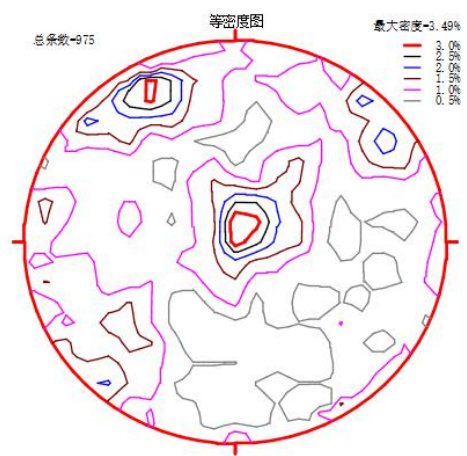
图 2-9 结构面等密度图
