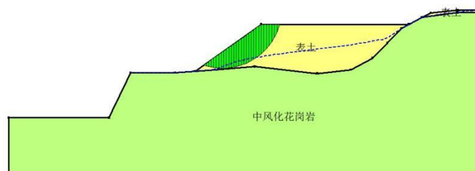
图 3-6 表土周转场不同工况下最危险滑弧示意图
