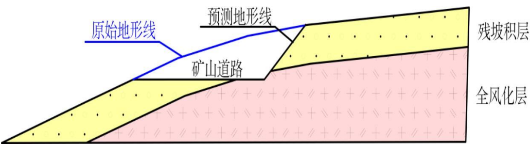
图 3-3 山坡露天开采时矿山公路边坡剖面示意图
