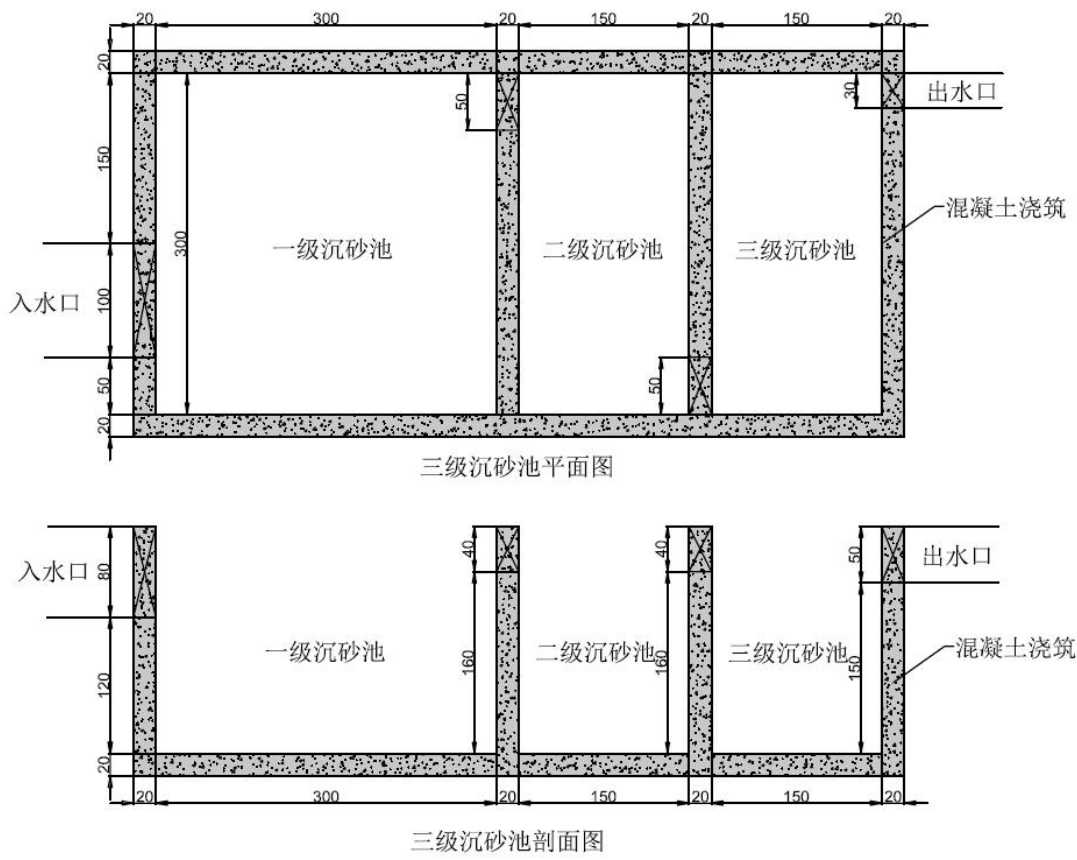
图 5-17 沉砂池工程大样图
