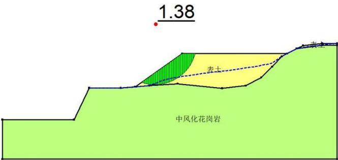
自然工况 Bishop 法计算结果
