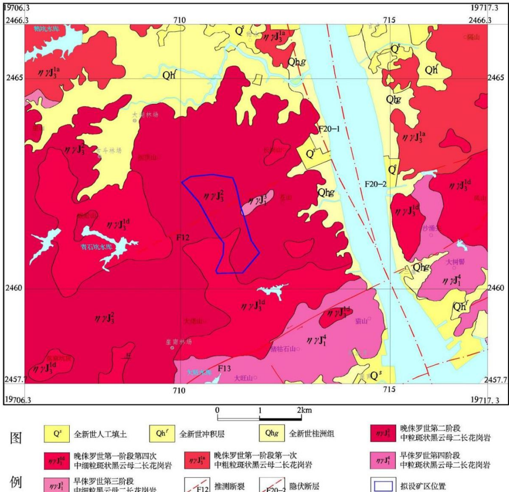
图 2-8 区域地质图(据 1:5 万新会区城市地质调查报告)
