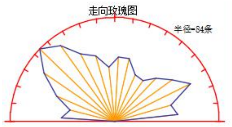
图 2-10 结构面走向玫瑰花图
