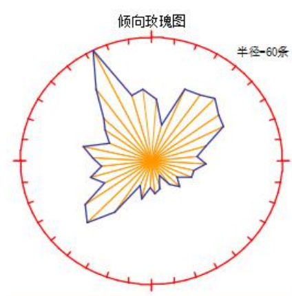
图 2-11 结构面倾向玫瑰花图
