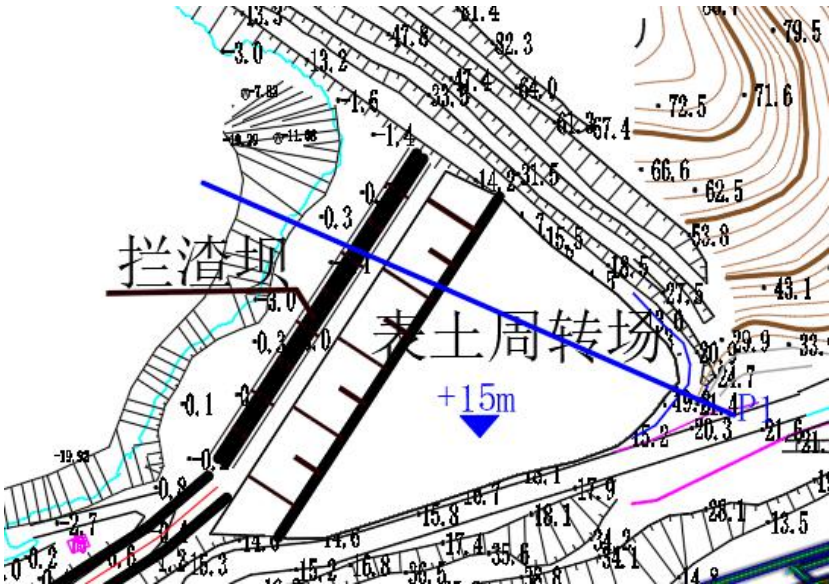
图 3-5 表土周转场边坡稳定性分析典型剖面平面图
