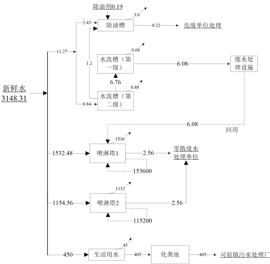
图 2-2 项目年水平衡图（单位：吨/年）
