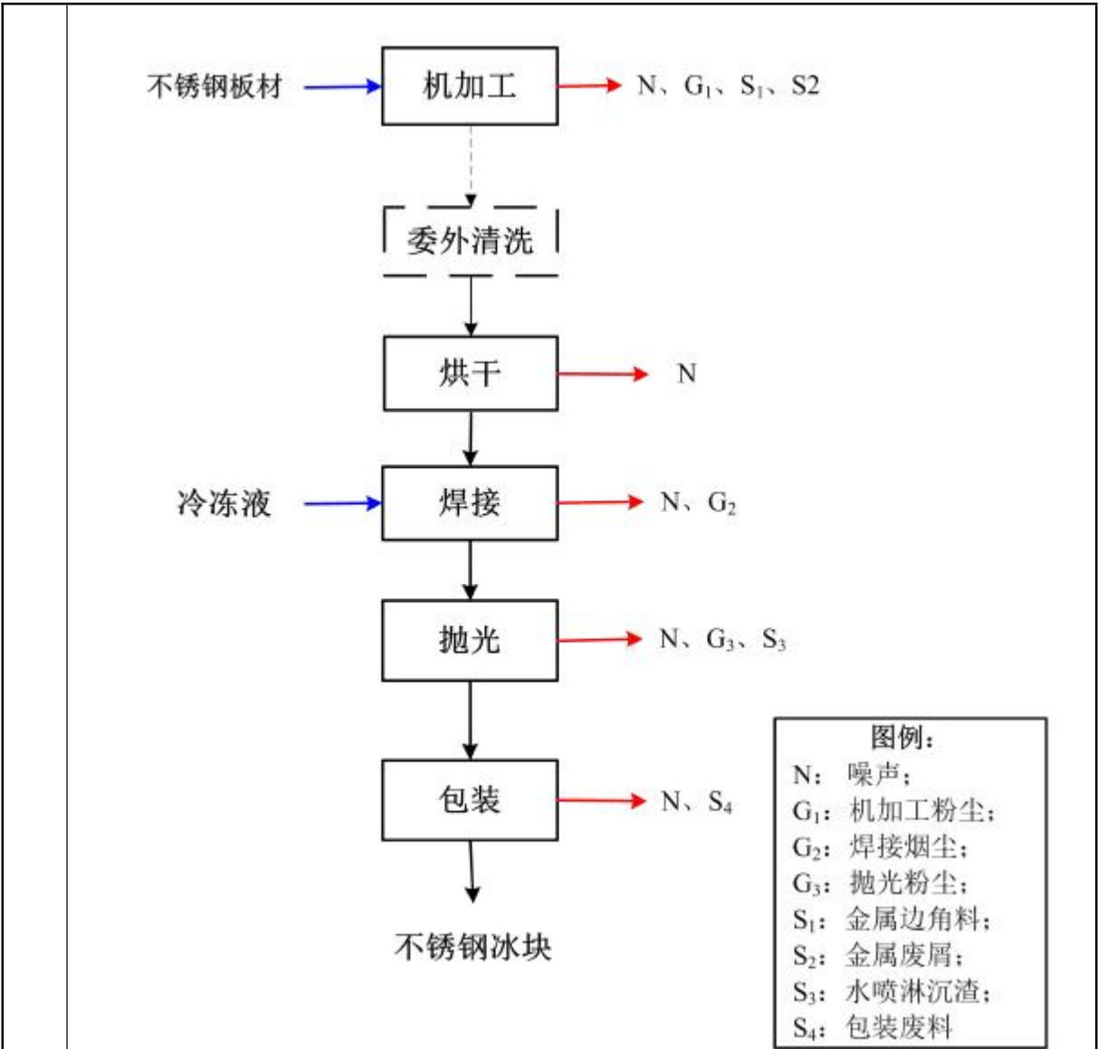
图 2-4 现有项目生产工艺流程图
