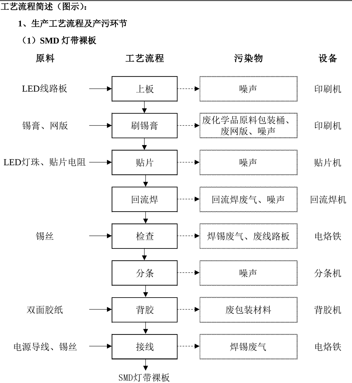
图2 SMD 灯带裸板生产工艺流程图
