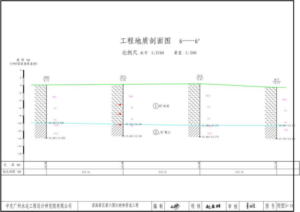
图 3.3-3 工程地质剖面图（节选）
