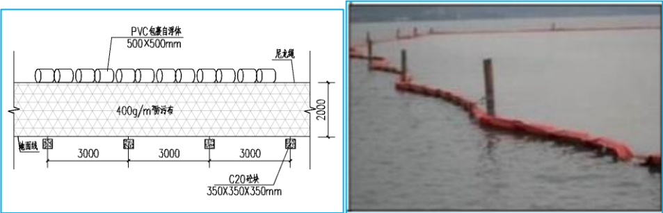
图 2.5-1 拦污帘示意图
