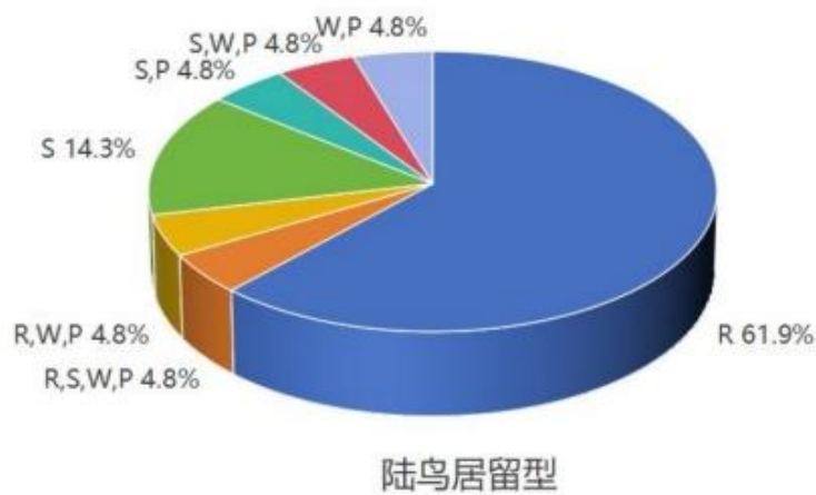
图 3.4-53 调查区域 2024 年 8 月陆鸟居留型组成
