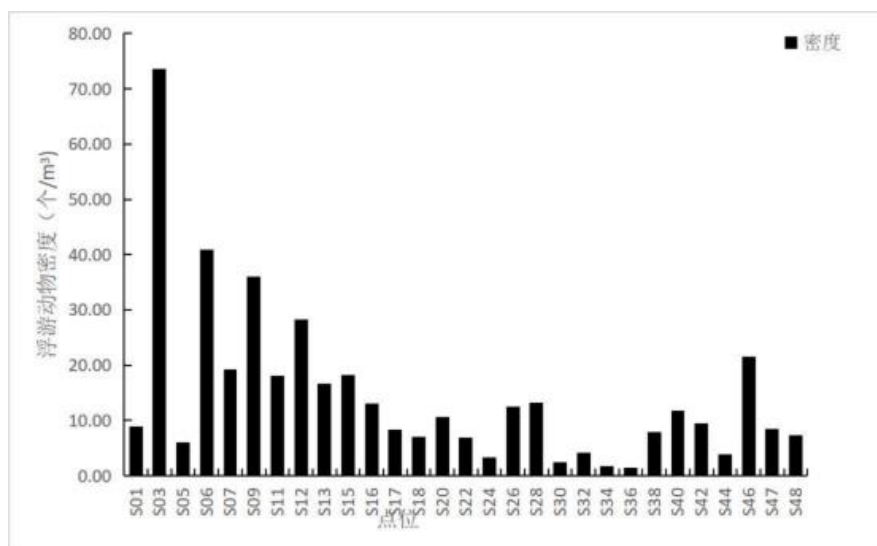
图 3.4-17 调查海域各点位浮游动物个体密度的分布图（单位：ind/ \text{m}^3 ）
