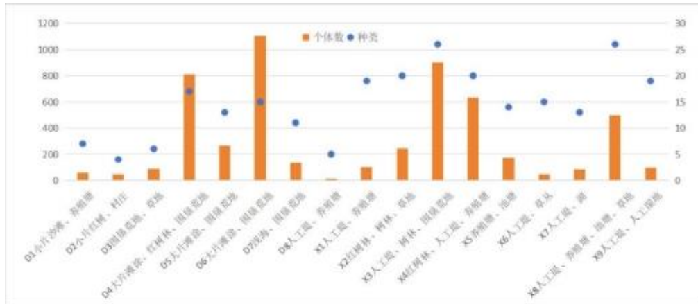
图 3.4-69 各样线、样点种类数和个体数
