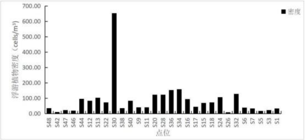
图 3.4-14 调查海域各点位浮游植物细胞密度分布图 (单位: \times 10^4 \text{ cells/m}^3 )
