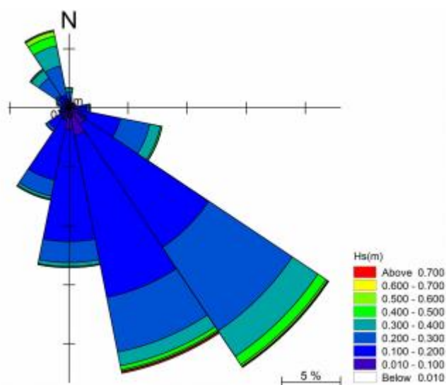
图 3.1-4 黄茅海临时波浪测站有效波高频率分布玫瑰图 (2018.7.10~2019.7.10)
