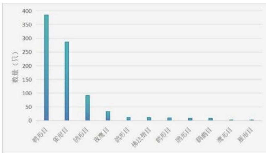
图 3.4-49 调查区域 2024 年 8 月各目鸟类数量
