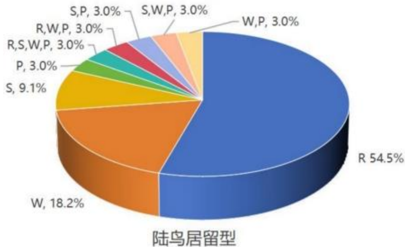
图 3.4-67 调查区域 2024 年年度陆鸟居留型组成
