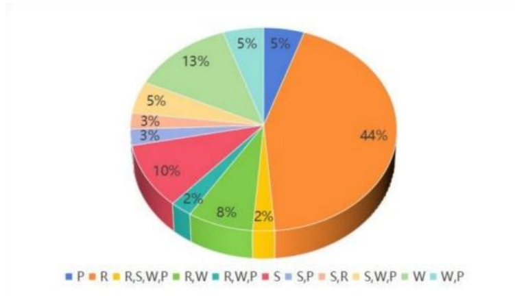
图 3.4-51 调查区域 2024 年 8 月鸟类居留型组成
