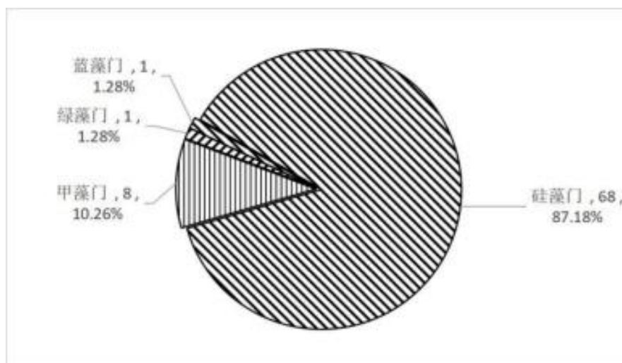
图 3.4-12 调查海域浮游植物种类组成图
