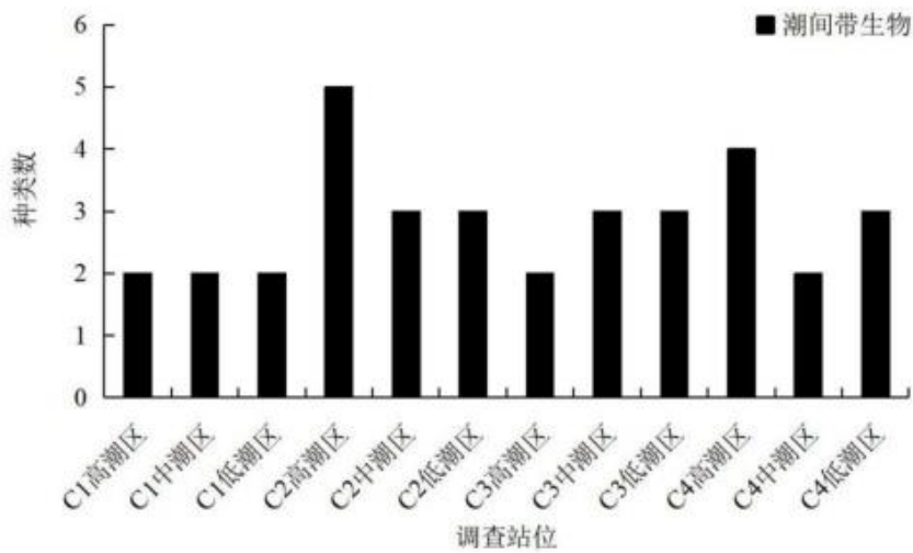
图 3.4-21 各调查站位潮间带生物种类分布图
