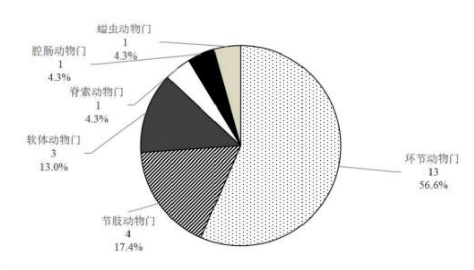
图 3.4-19 调查海域底栖生物的种类组成
