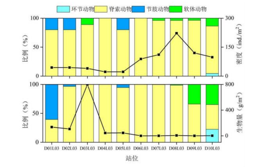
图 3.4-43 各站位大型底栖动物栖息密度与生物量
