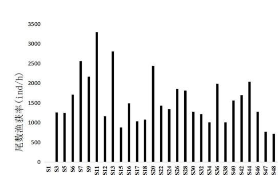
图 3.4-27 各站位总尾数渔获率分布
