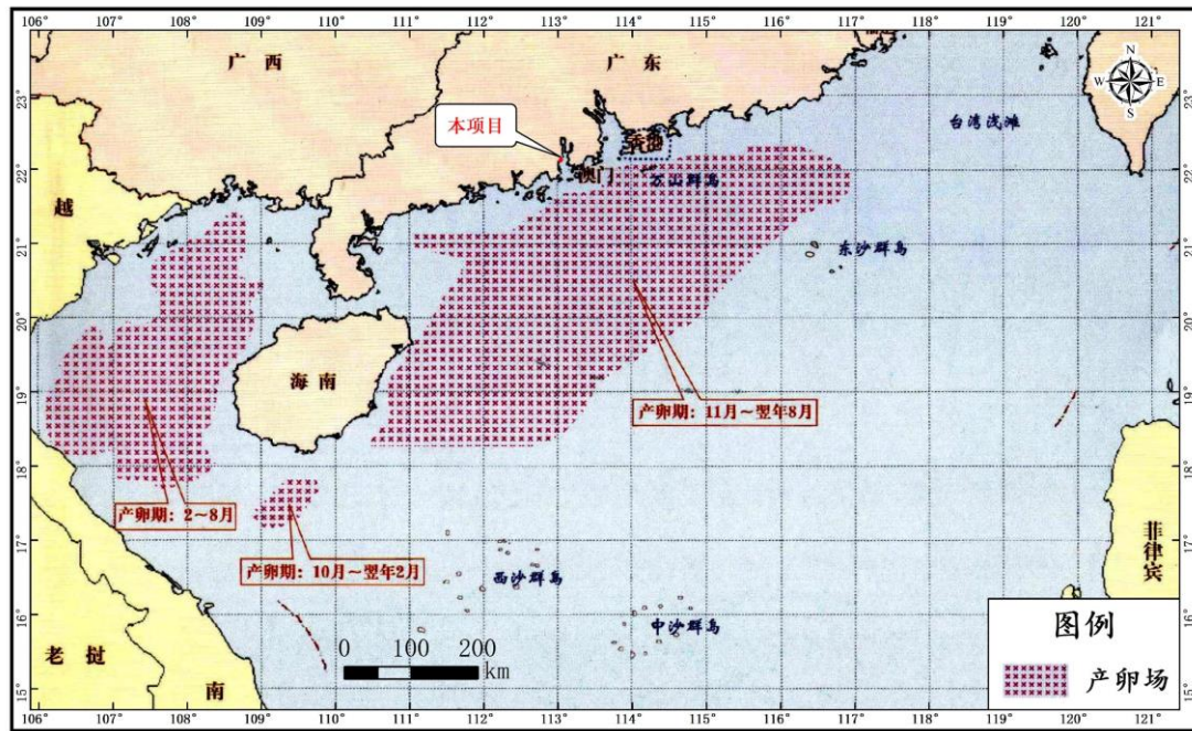
图 3.3-3 南海底层、近底层鱼类产卵场示意图
